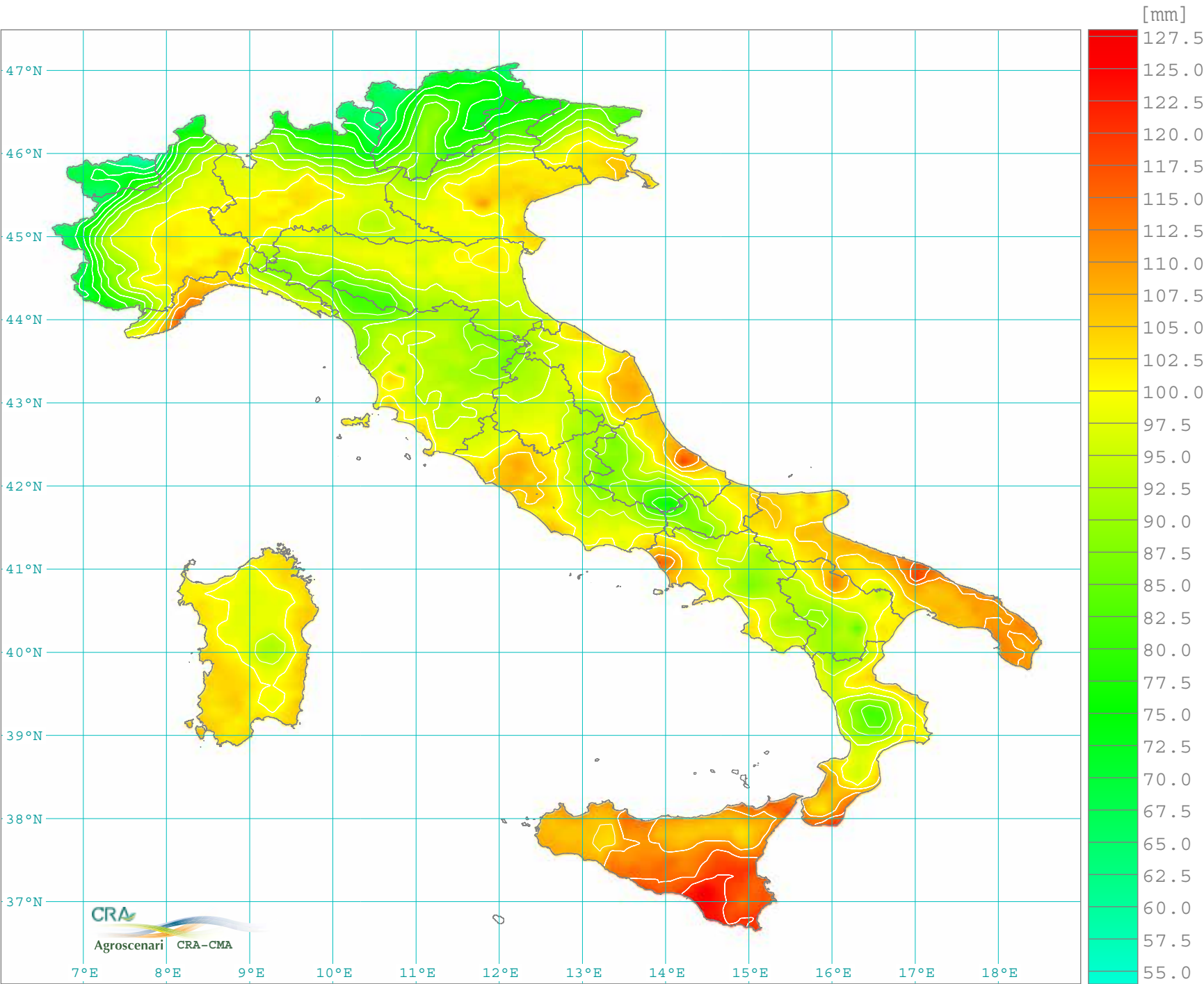
Evapotraspirazione potenziale totale giugno (1961-1990)
