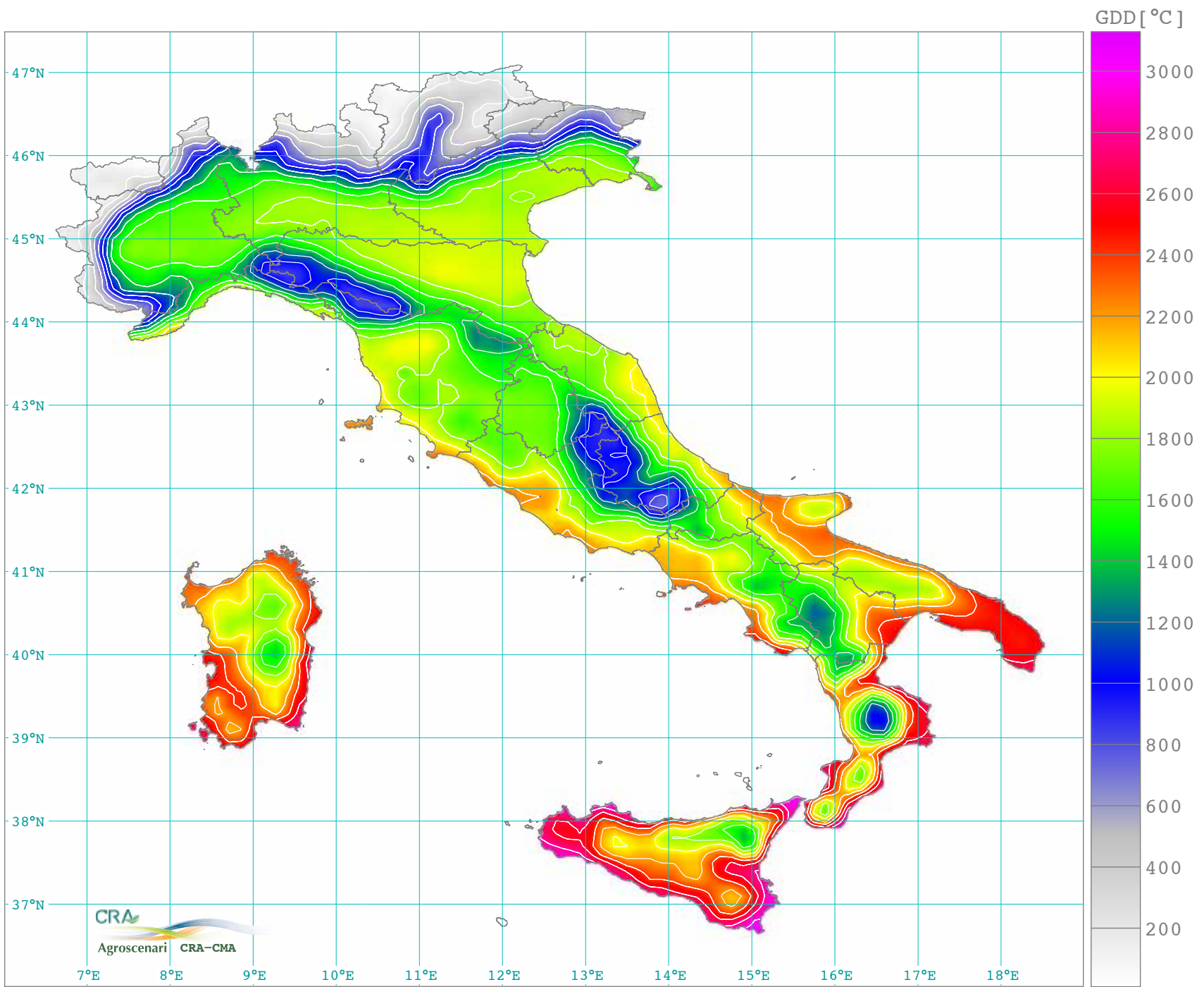
Sommatorie termiche annue soglia 10 °C (1961-1990)
