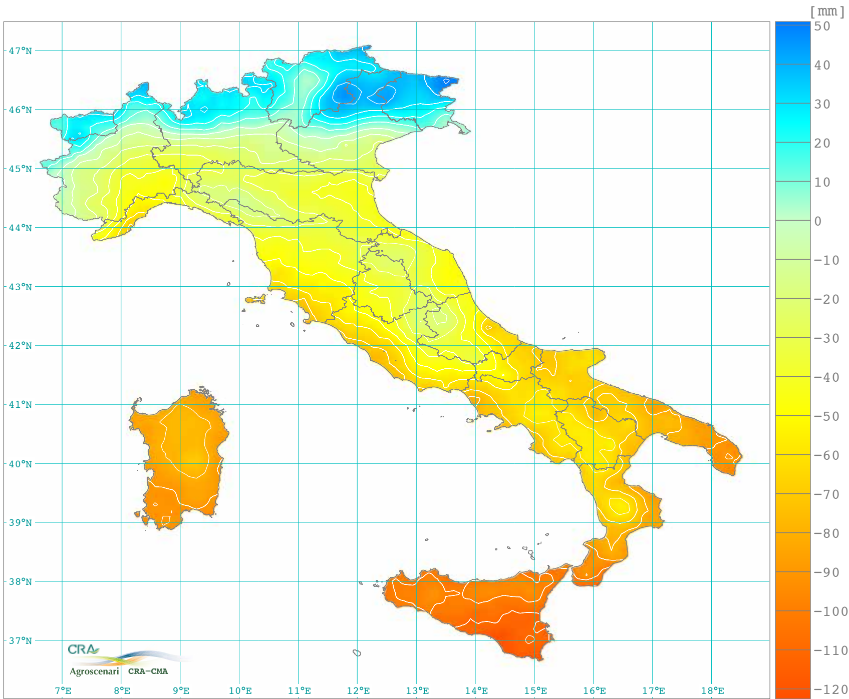
Bilancio idroclimatico mensile giugno (1961-1990)
