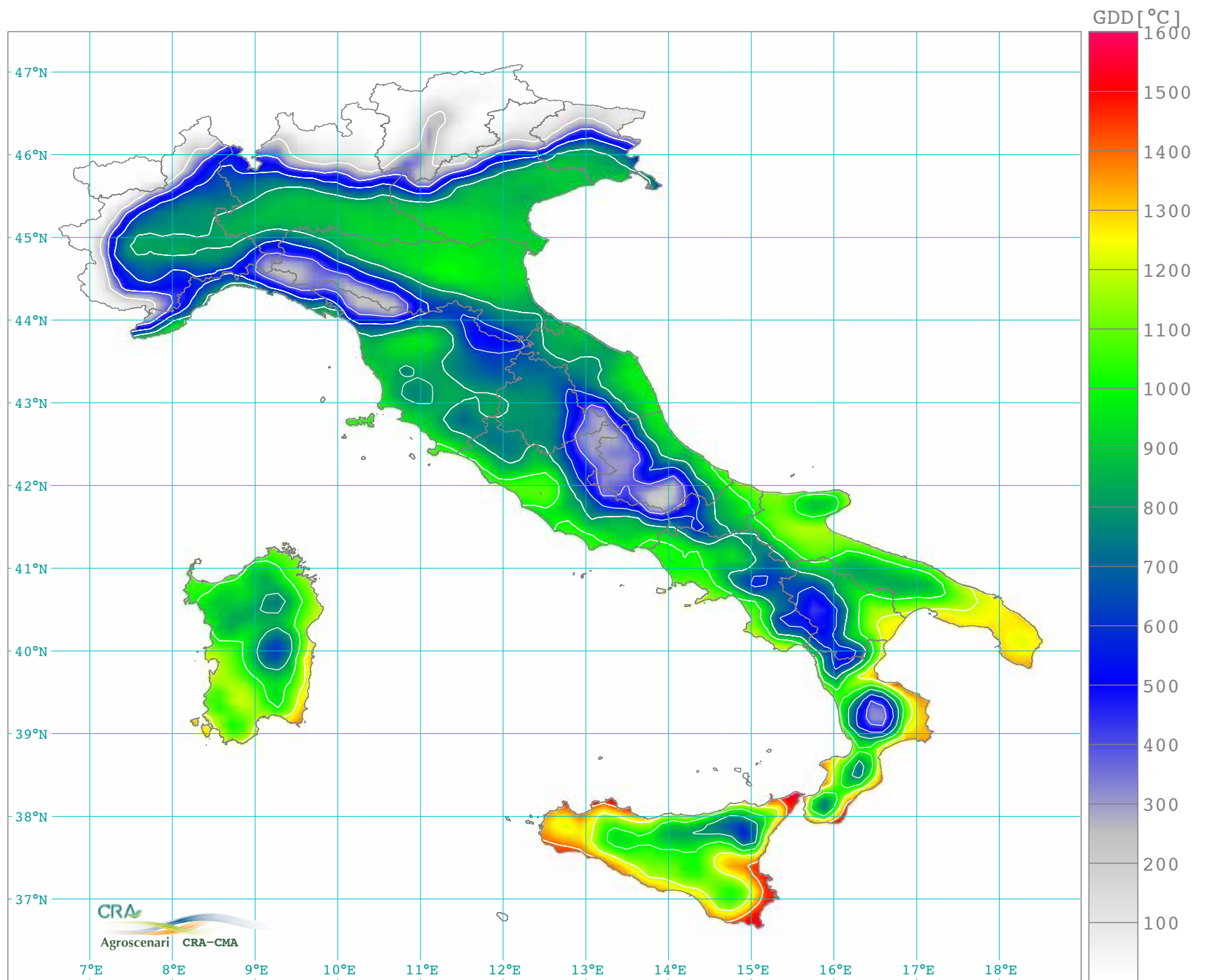
Sommatorie termiche annue soglia 15 °C (1961-1990)
