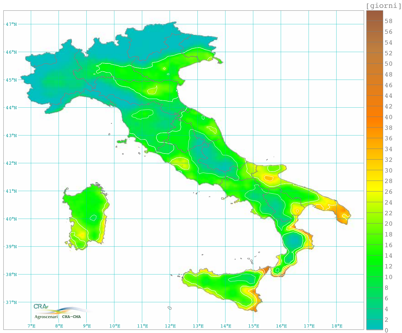
Numero medio annuo di giorni con temperatura massima > 30 °C (1961-1990)
