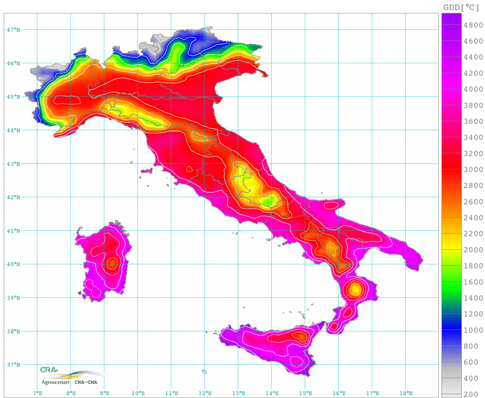
Sommatorie termiche annue soglia 5 °C (1961-1990)
