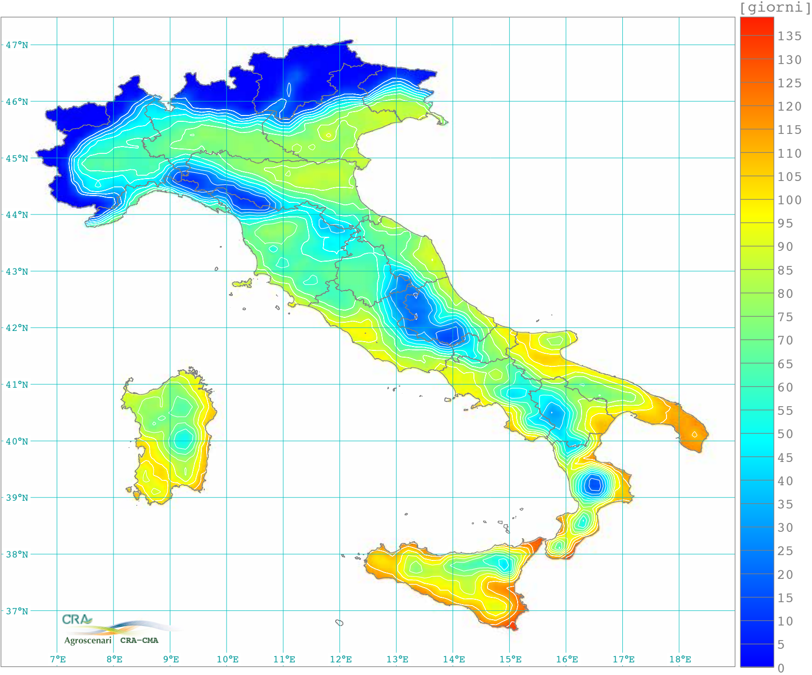
Numero medio annuo di giorni estivi (1961-1990)
