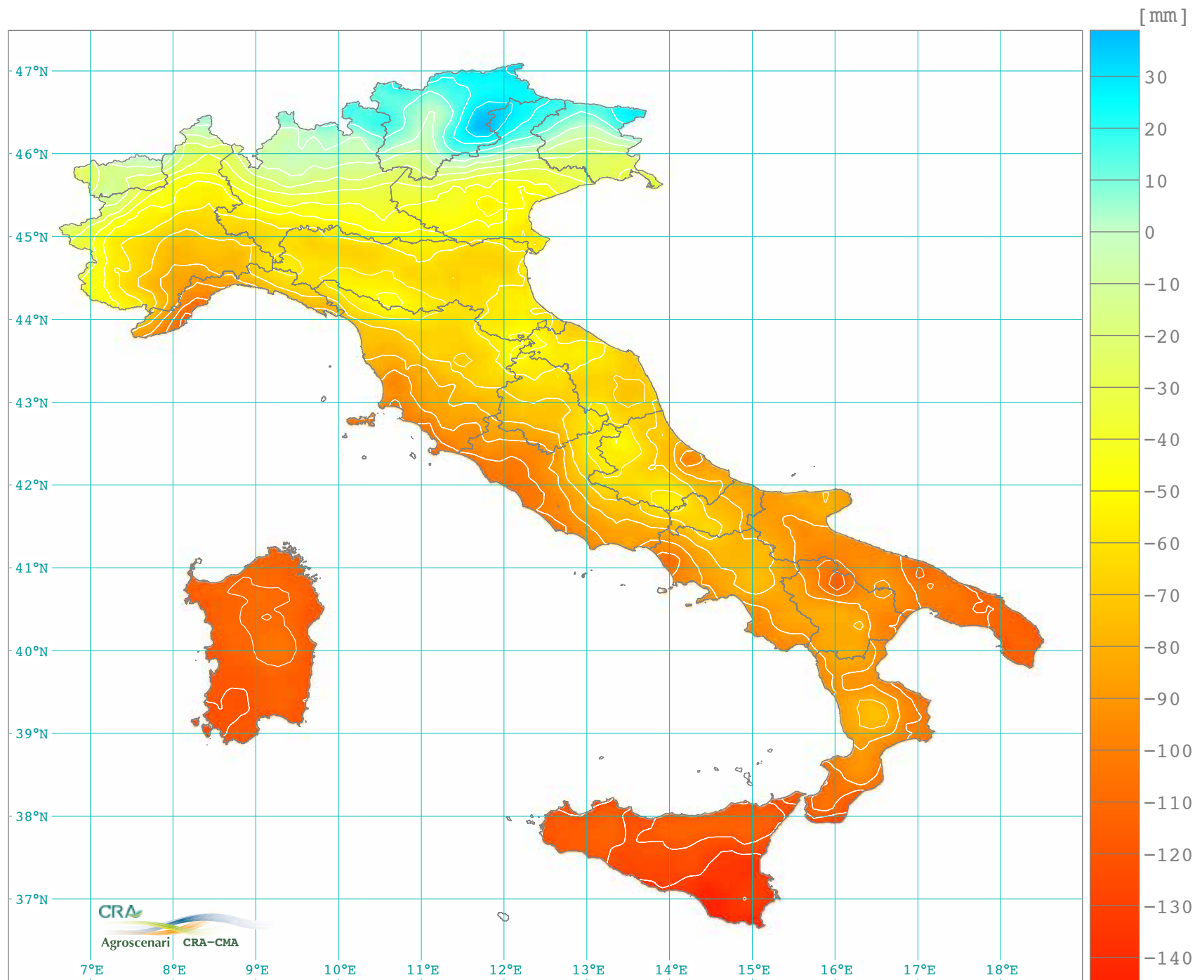
Bilancio idroclimatico mensile luglio (1961-1990)
