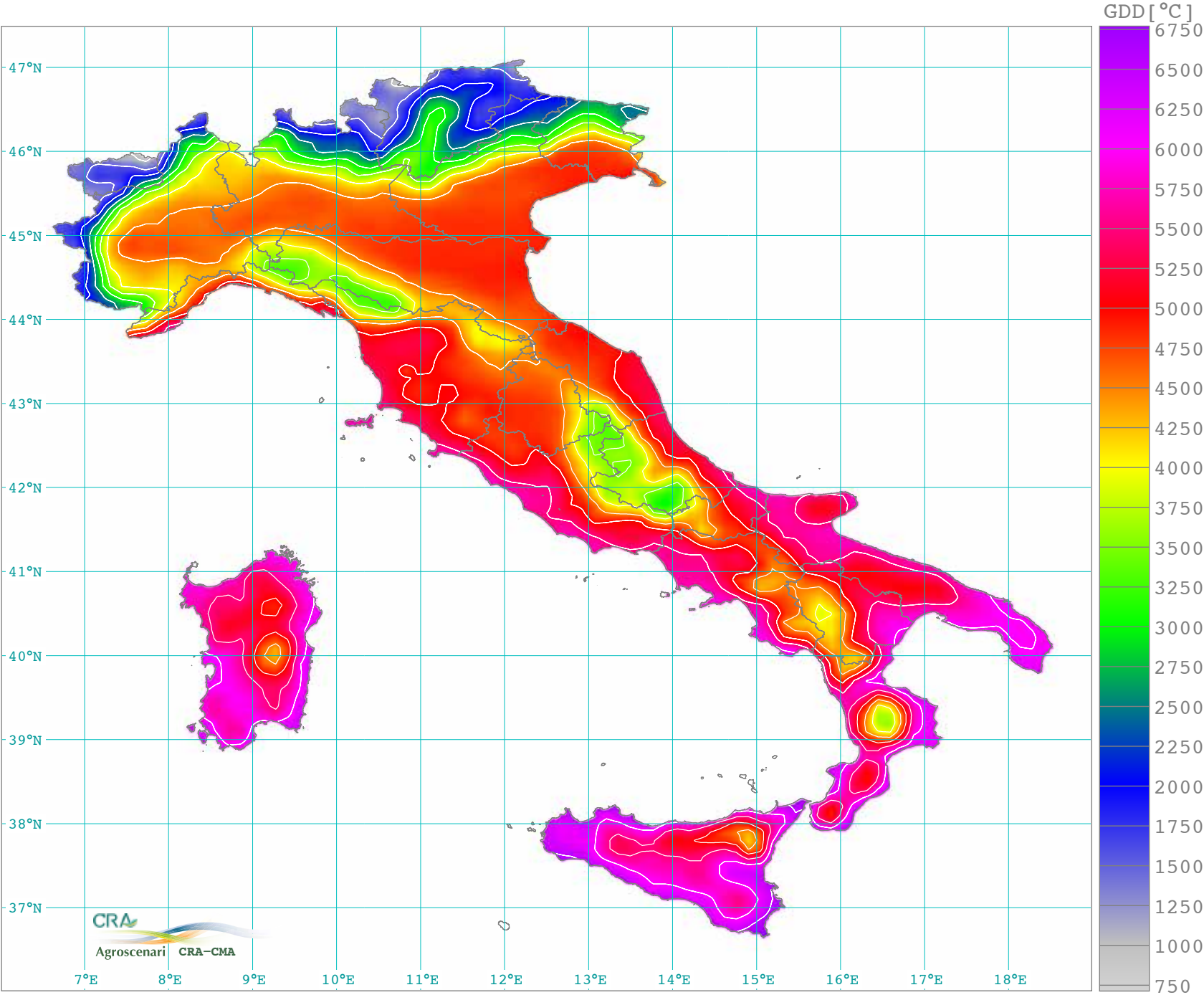
Sommatorie termiche annue soglia 0 °C (1961-1990)
