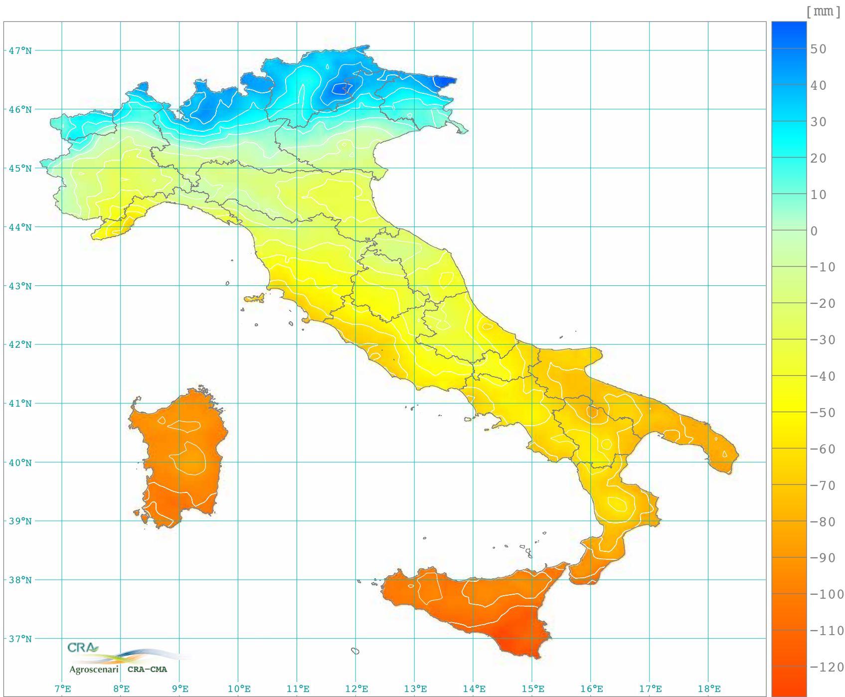
Bilancio idroclimatico mensile agosto (1961-1990)
