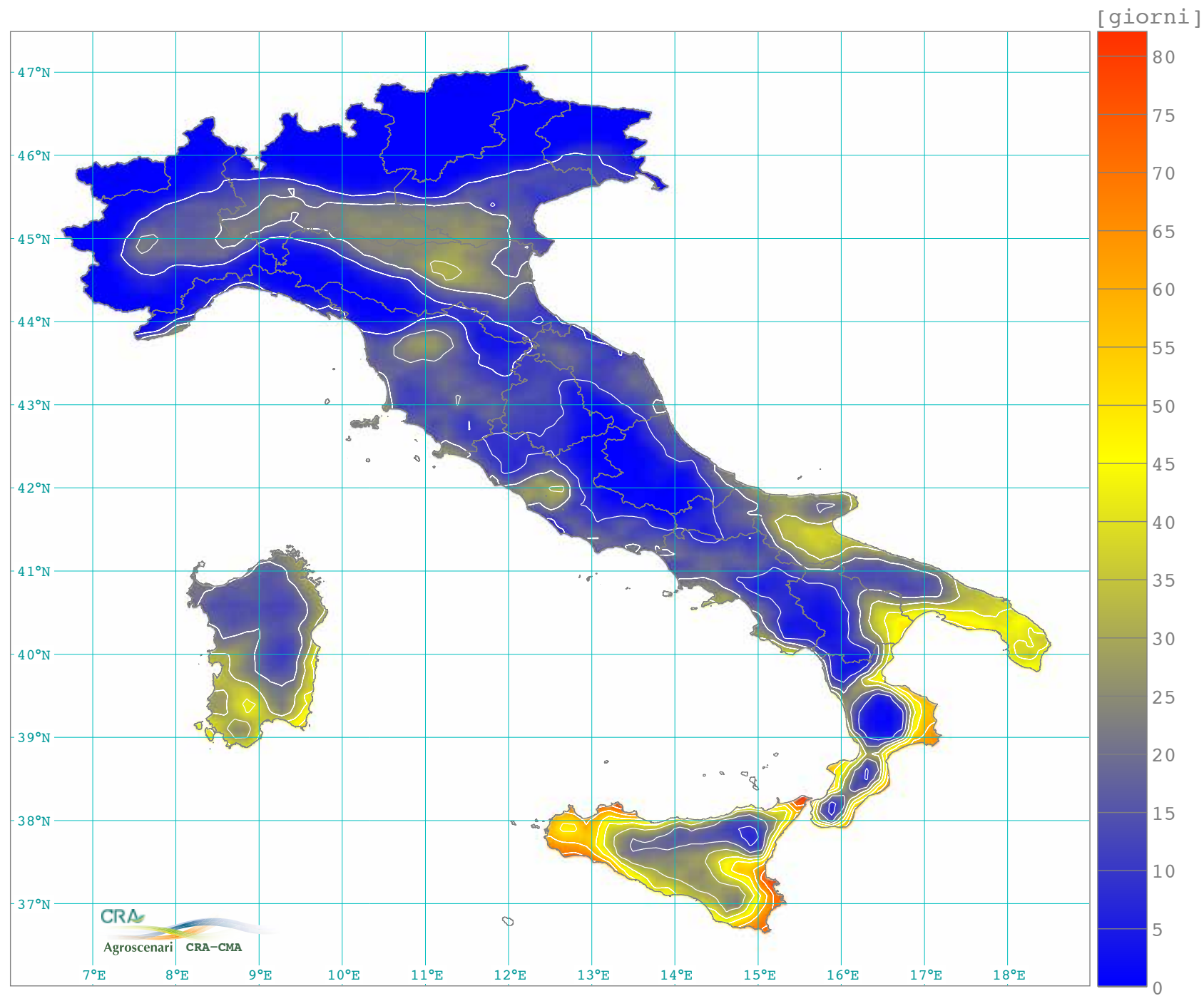
Numero medio annuo di notti tropicali (1961-1990)
