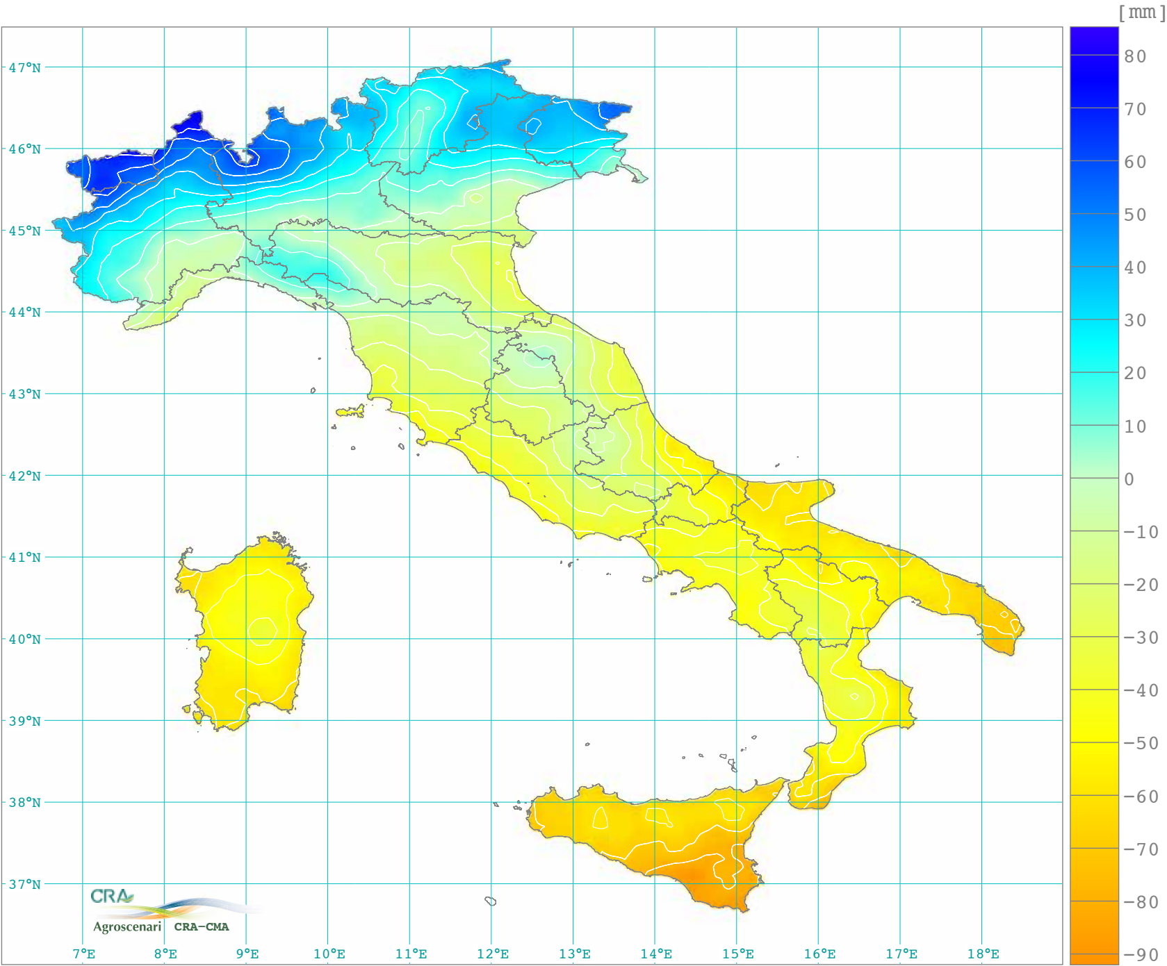
Bilancio idroclimatico mensile maggio (1961-1990)
