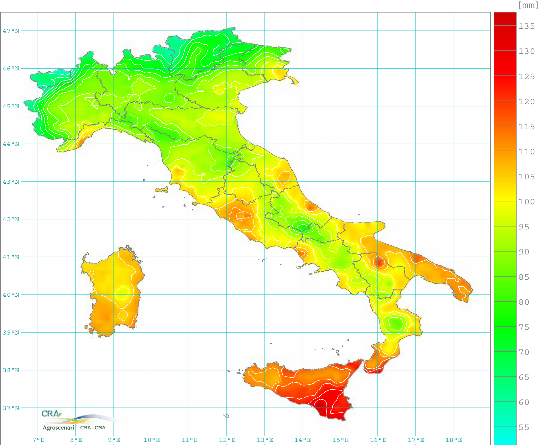
Evapotraspirazione potenziale totale agosto (1961-1990)
