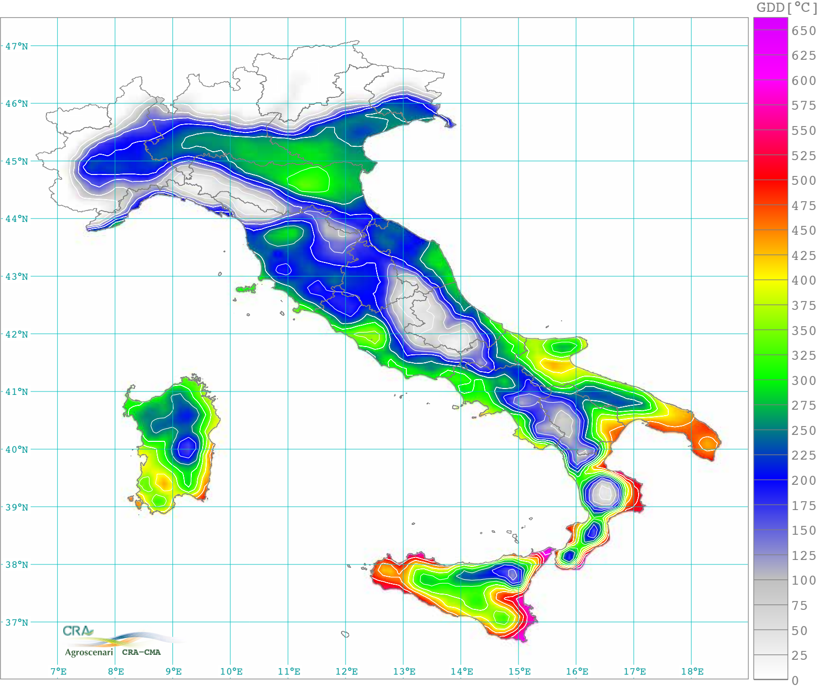
Sommatorie termiche annue soglia 20 °C (1961-1990)
