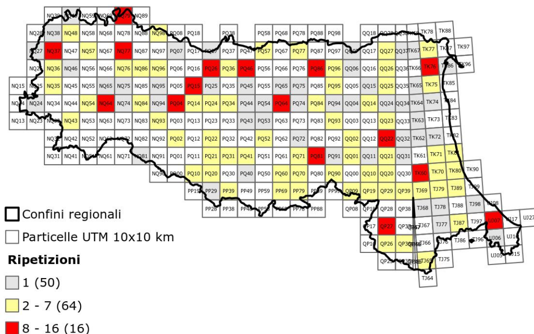
Figura 1.2: Particelle UTM 10x10 km utilizzate nel calcolo degli andamenti delle specie tipiche di ambiente agricolo e dell'andamento del Farmland Bird Index: le particelle sono distinte in base al numero di ripetizioni annuali (in rosso le particelle visitate almeno 8 anni, in giallo quelle visitate un numero inferiore di anni). In grigio sono riportate le particelle con almeno sette stazioni censite solamente una volta durante il periodo 2000-2017, dunque ancora non utilizzate nel calcolo degli andamenti.
