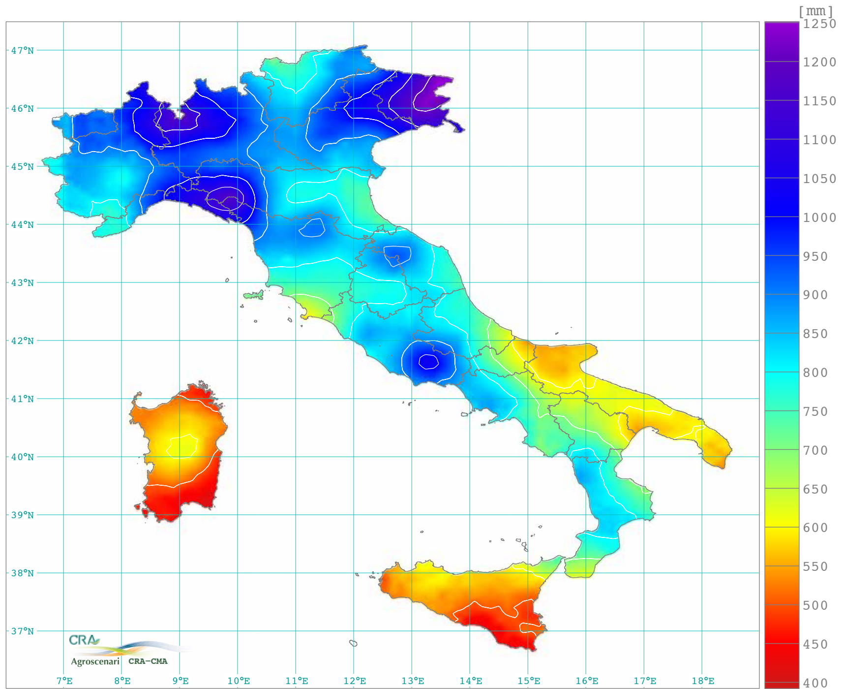
Precipitazione totale annua (1971-2000)
