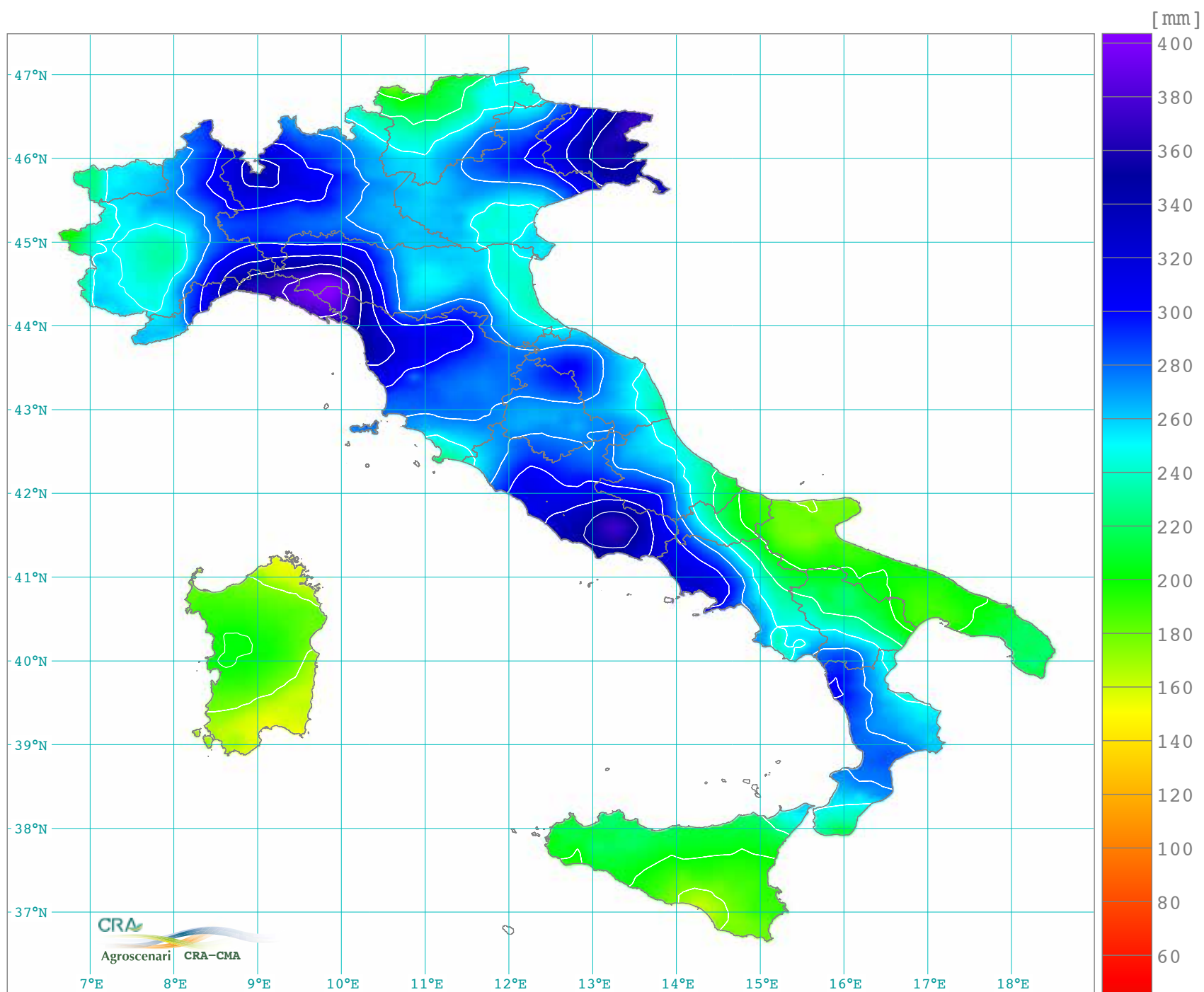
Precipitazione totale stagionale autunno: settembre, ottobre e novembre (1971-2000)
