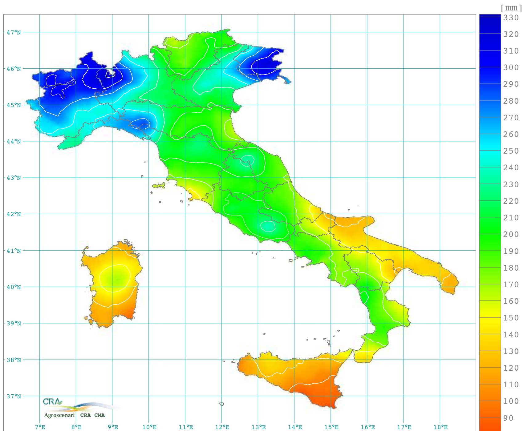
Precipitazione totale stagionale primavera: marzo, aprile e maggio (1971-2000)
