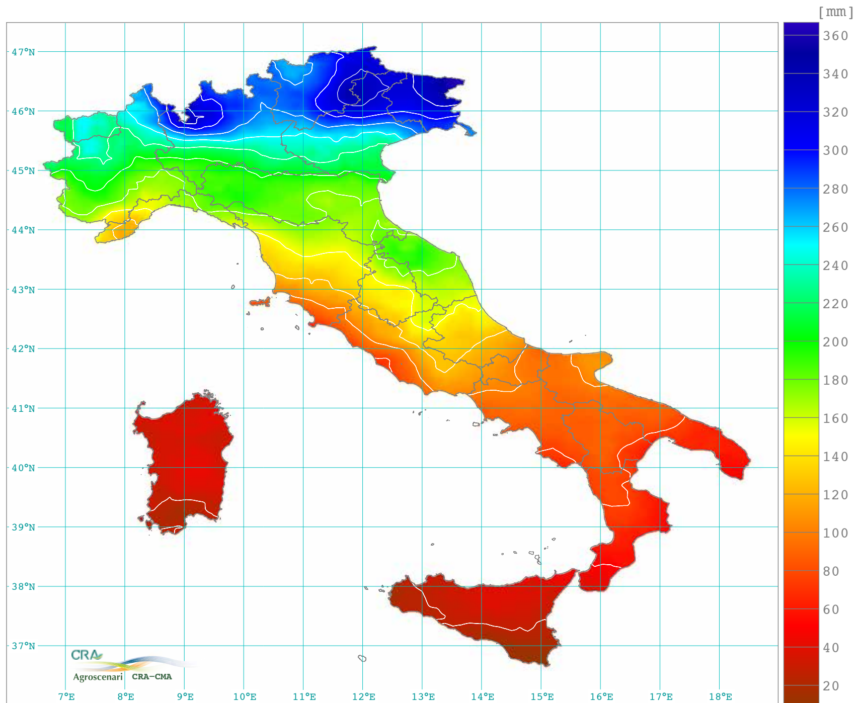
Precipitazione totale stagionale estate: giugno, luglio e agosto (1971-2000)
