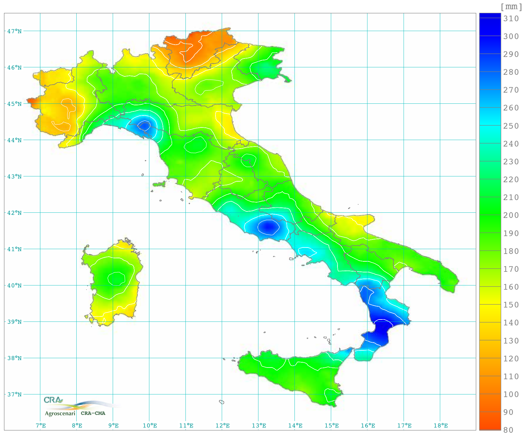
Precipitazione totale stagionale inverno: dicembre, gennaio e febbraio (1971-2000)
