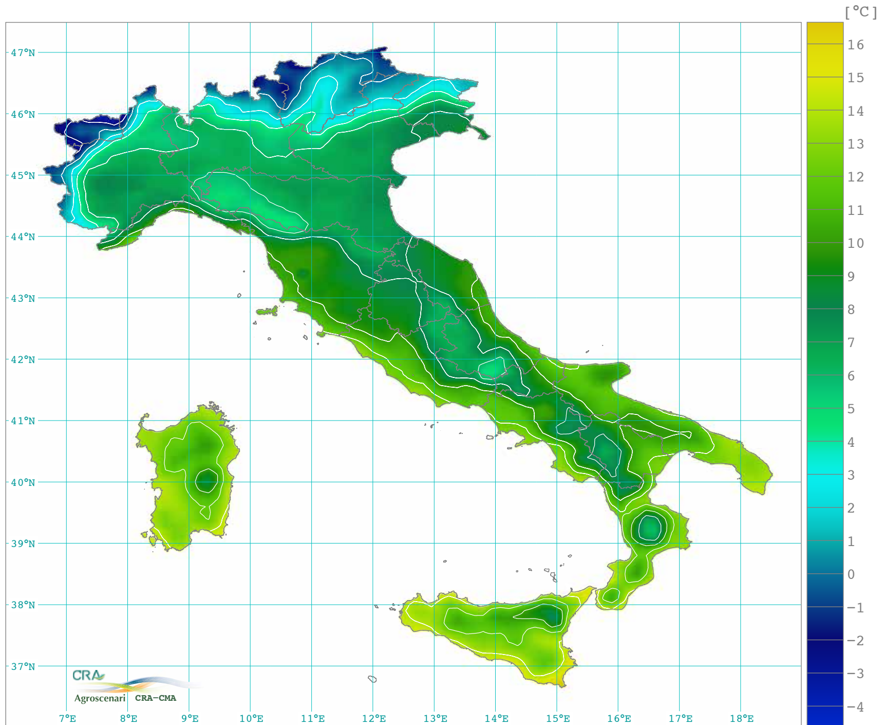
Temperatura massima media stagionale inverno: dicembre, gennaio e febbraio (1971-2000)
