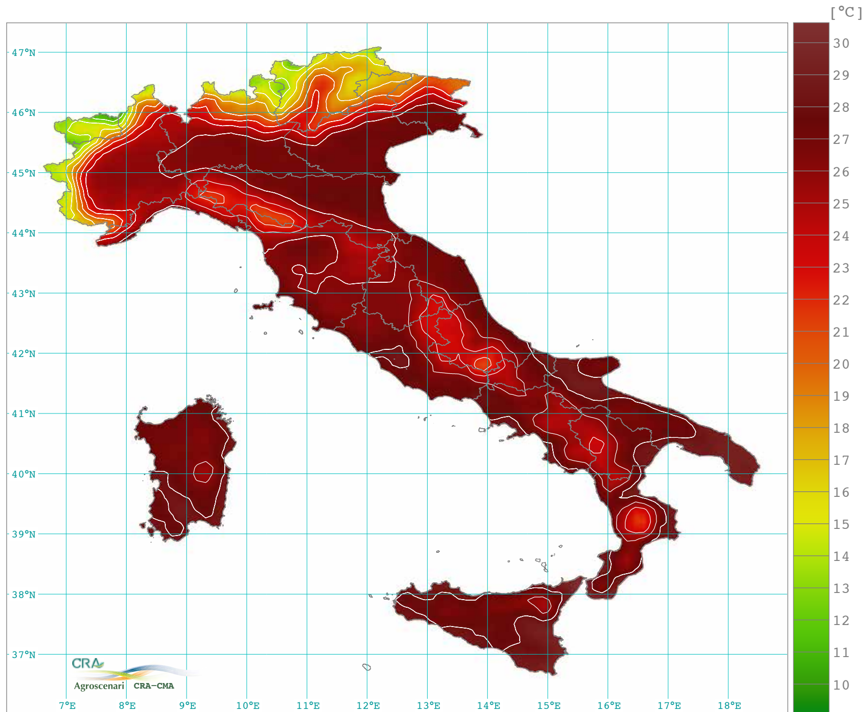
Temperatura massima media stagionale estate: giugno, luglio e agosto (1971-2000)
