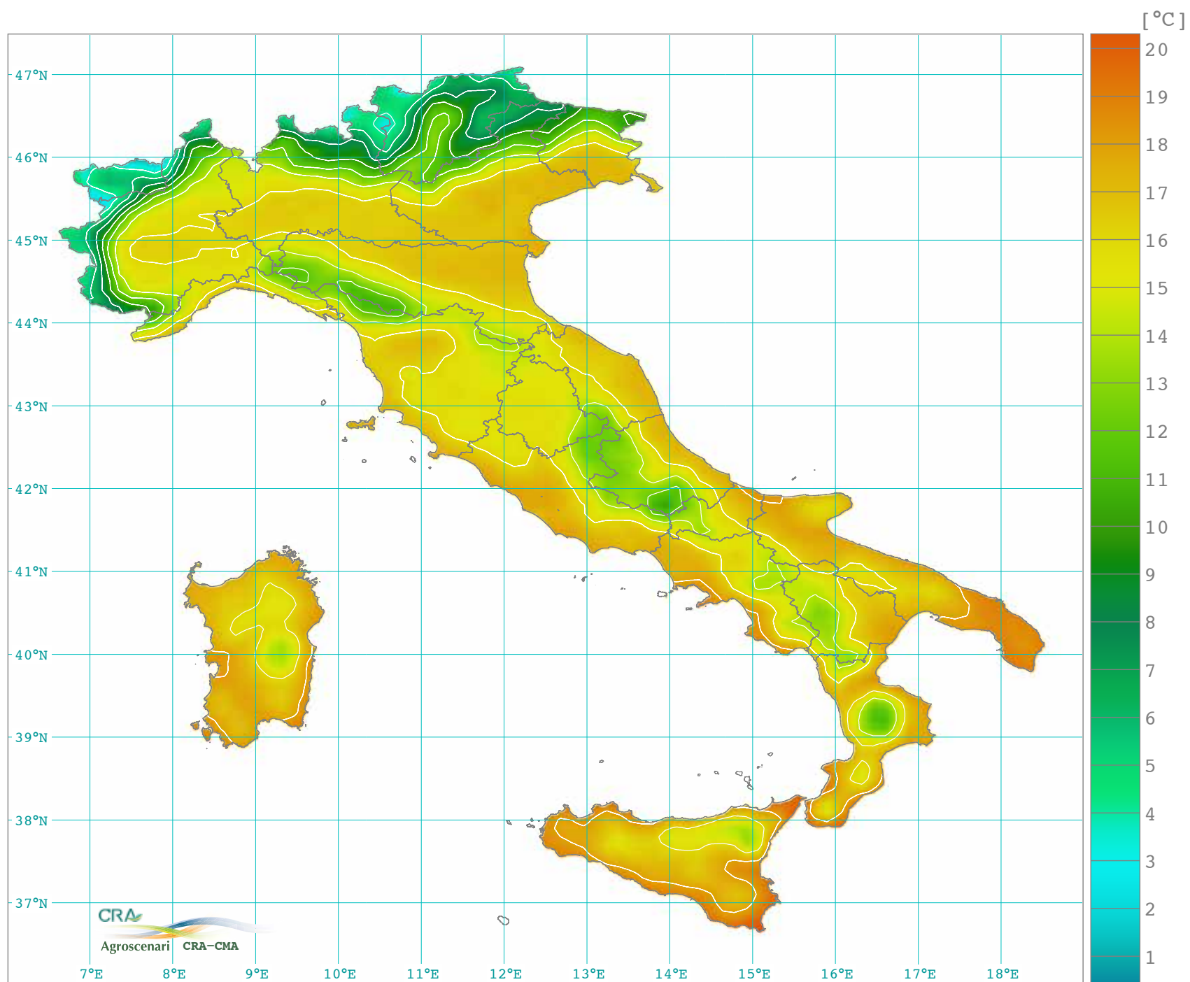
Temperatura massima media stagionale primavera: marzo, aprile e maggio (1971-2000)
