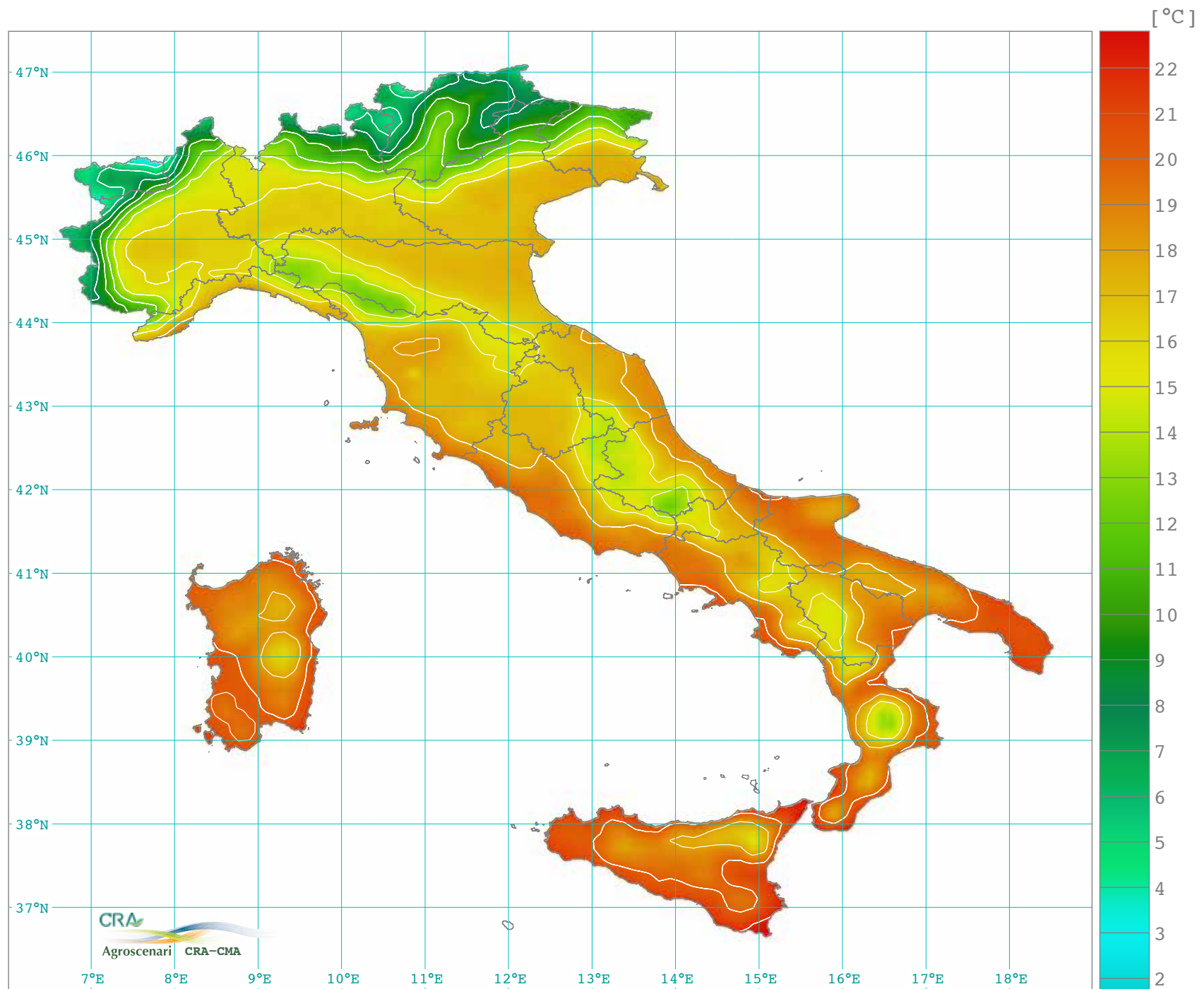
Temperatura massima media annua (1971-2000)
