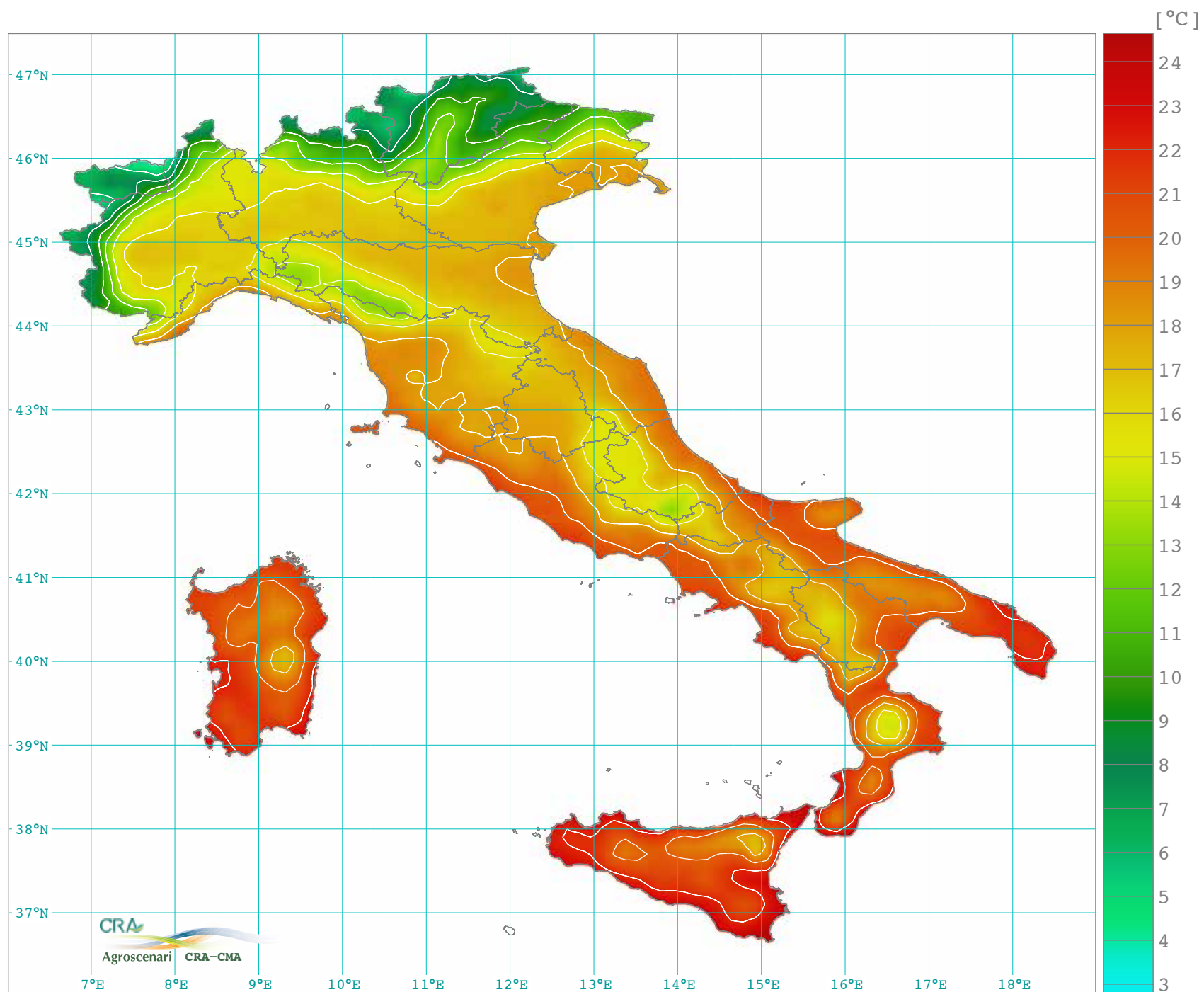
Temperatura massima media stagionale autunno: settembre, ottobre e novembre (1971-2000)
