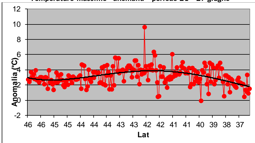
Fig. 6 - Diagramma latitudinale delle anomalie delle temperature massime nel periodo in esame. Latitudinal diagram of anomaly of maximum temperature for the analysed period
