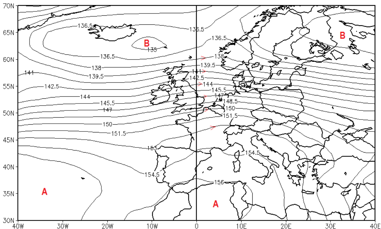
Fig. 1 - Topografia media del livello di pressione di 850 hPa (in media 1.5 km di quota) per il periodo 21 - 28 giugno. Le frecce inserite danno un'idea orientativa della direzione e del verso del flusso, di cui considerano la sola componente geostrofica. Gli assi delle saccature sono in blu e quelli dei promontori in rosso.
