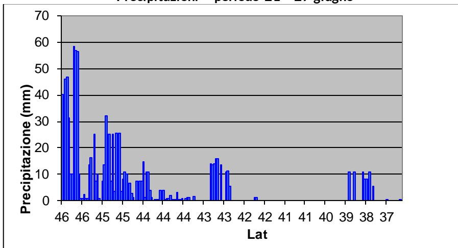
Fig. 5 - Diagramma latitudinale delle precipitazioni nel periodo in esame. Latitudinal diagram of precipitation for the analysed period
