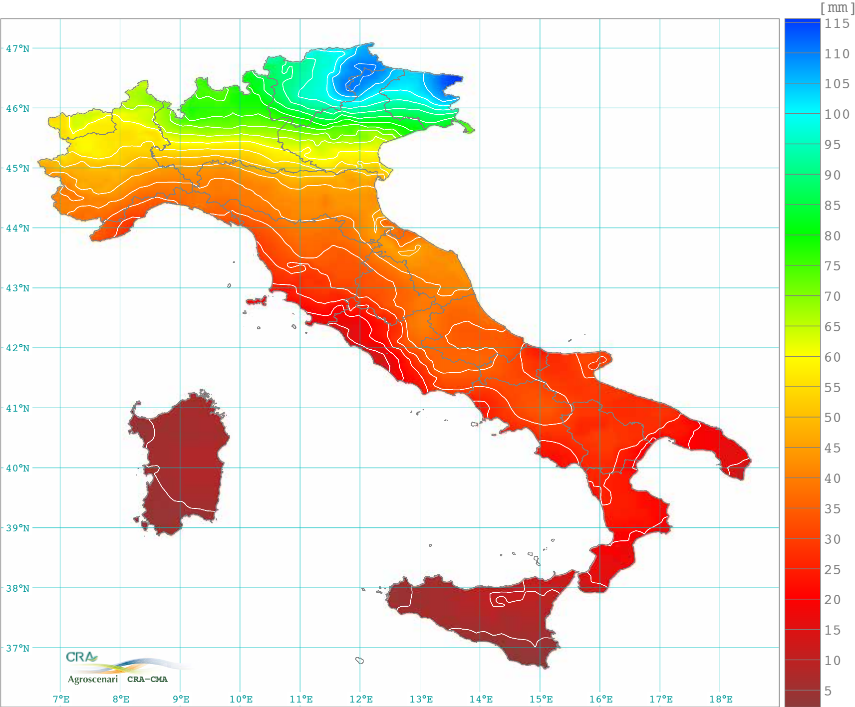
Precipitazione totale mensile luglio (1981-2010)
