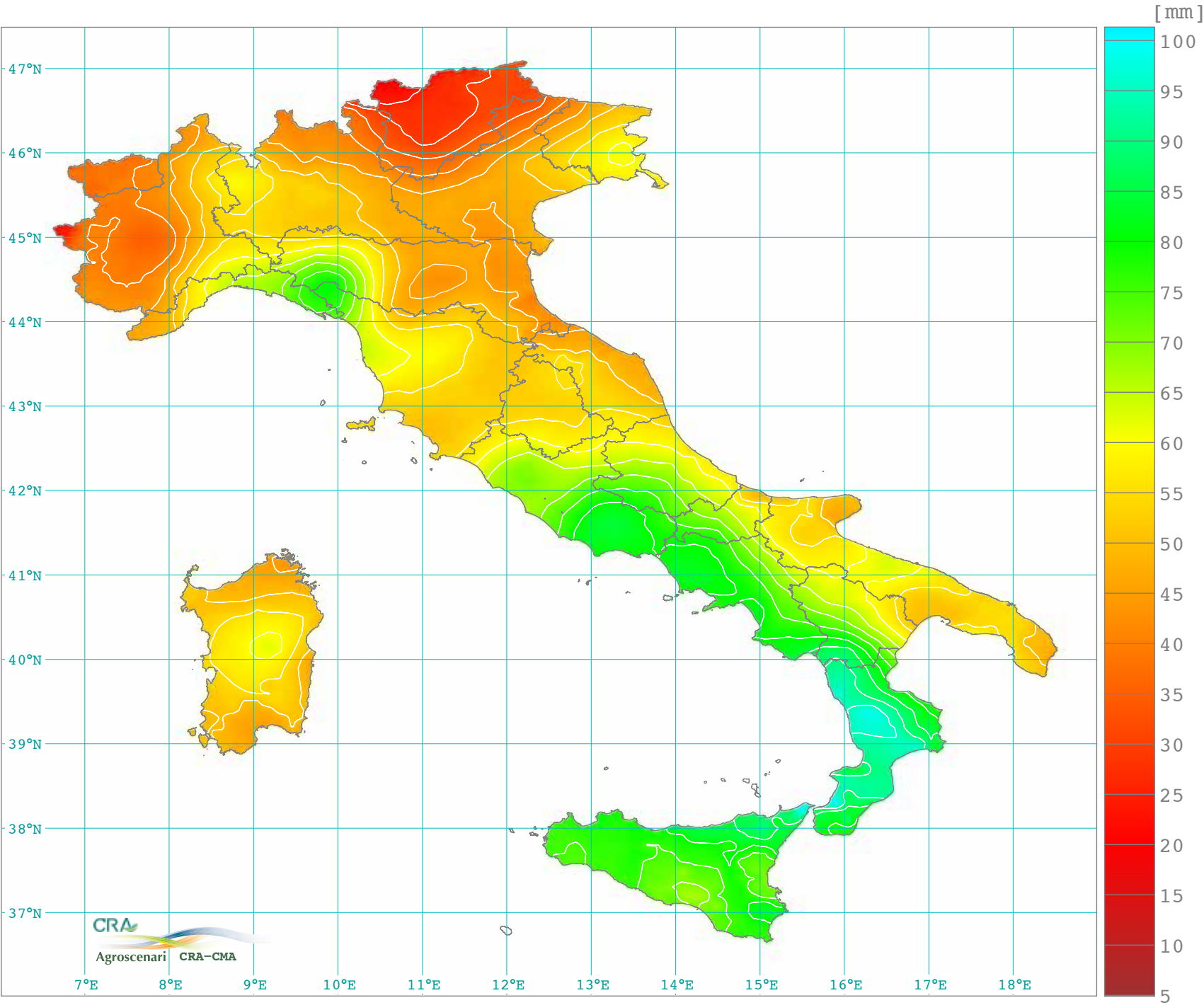
Precipitazione totale mensile gennaio (1981-2010)
