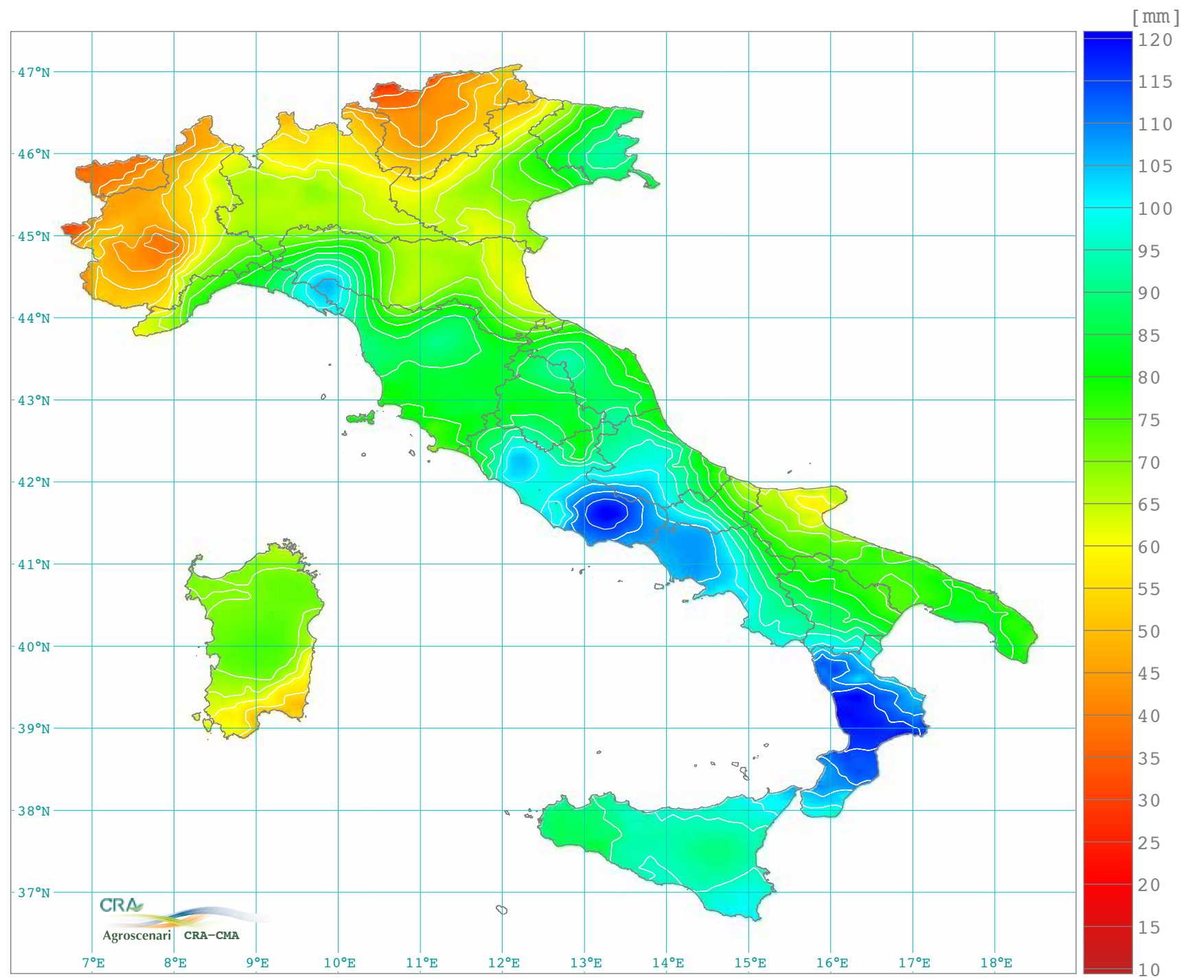
Precipitazione totale mensile dicembre (1981-2010)
