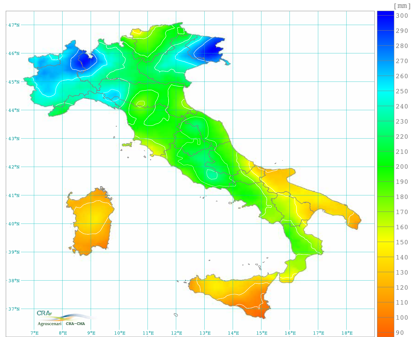
Precipitazione totale stagionale primavera: marzo, aprile e maggio (1981-2010)
