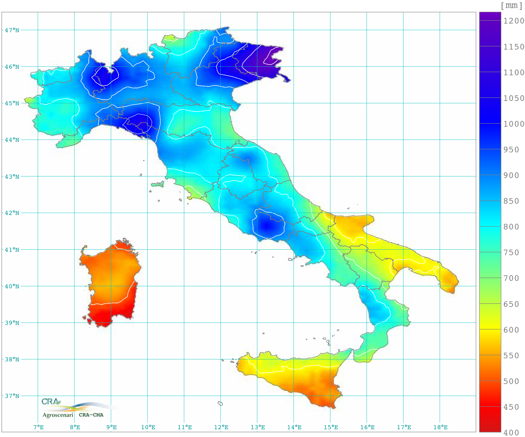
Precipitazione totale annua (1981-2010)
