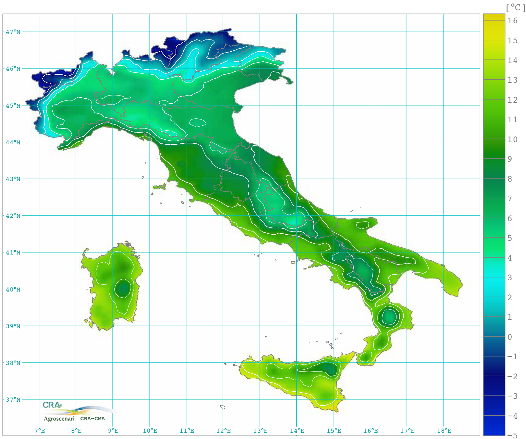
Temperatura massima media stagionale inverno: dicembre, gennaio e febbraio (1961-1990)
