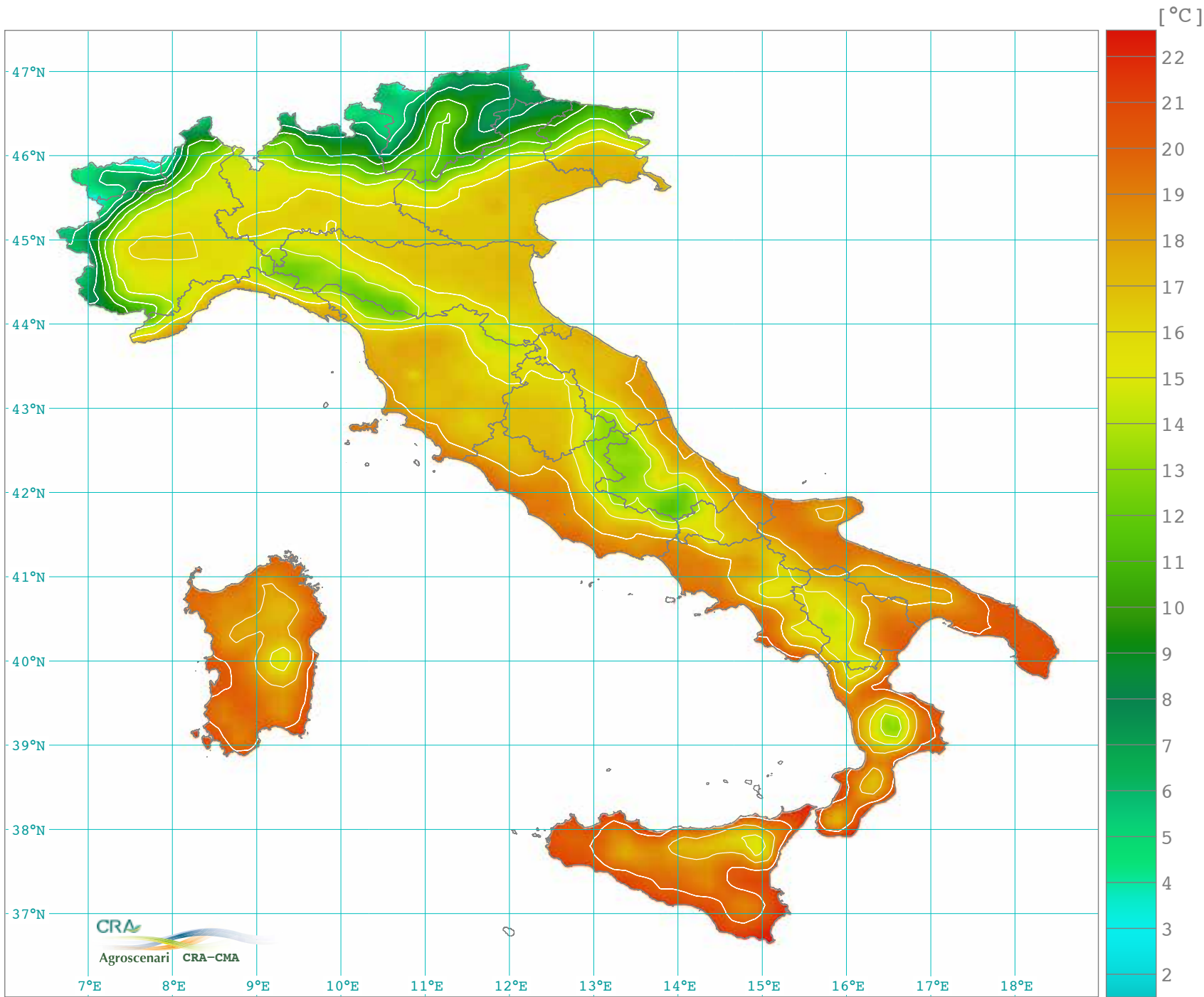
Temperatura massima media annua (1961-1990)
