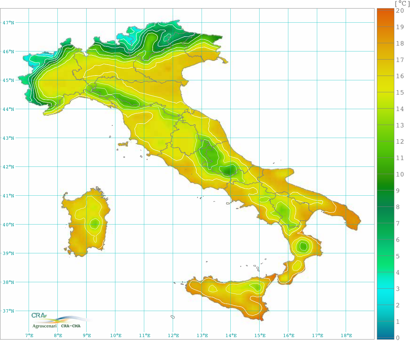
Temperatura massima media stagionale primavera: marzo, aprile e maggio (1961-1990)
