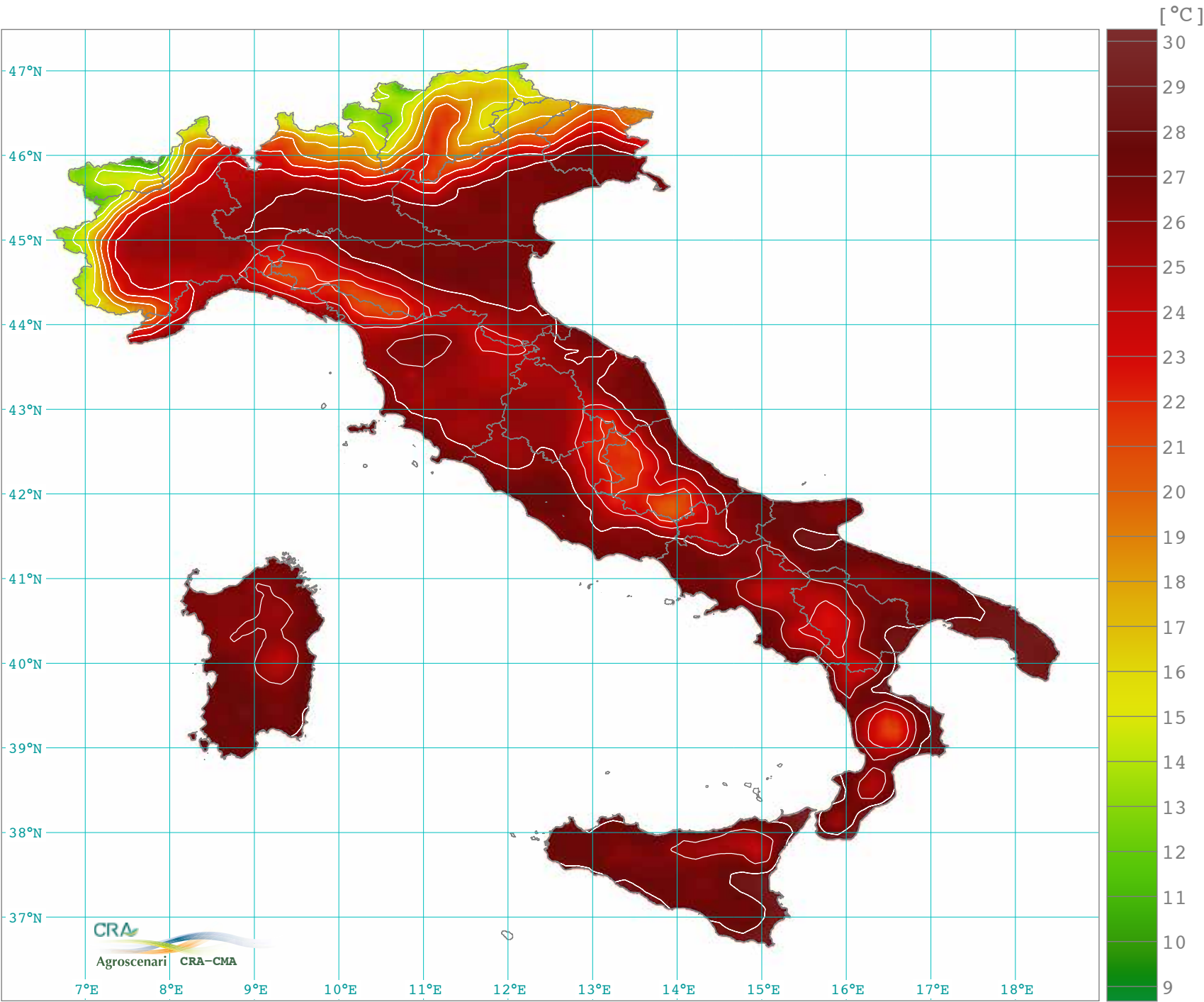
Temperatura massima media stagionale estate: giugno, luglio e agosto (1961-1990)
