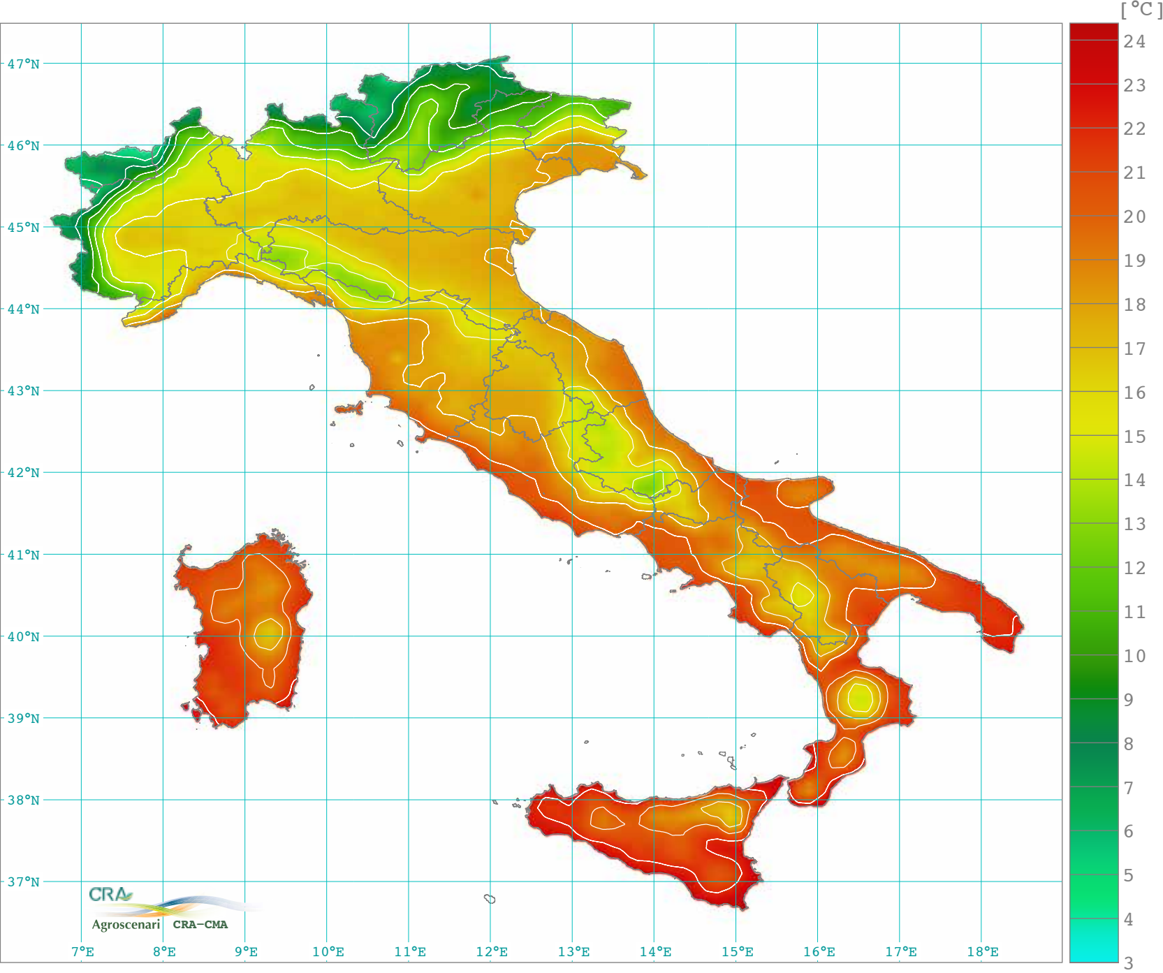
Temperatura massima media stagionale autunno: settembre, ottobre e novembre (1961-1990)
