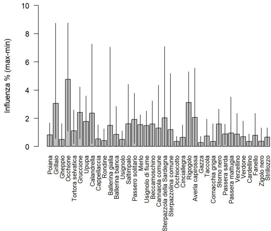
Figura 7. Sensitività del Farmland Bird Index al contributo delle singole specie. Per ogni specie è stata stimata la differenza percentuale in valore assoluto tra il Farmland Bird Index e l'indicatore ricalcolato senza considerare la specie stessa. Le colonne rappresentano i valori medi negli anni di indagine; le barre di errore il range dei valori.
