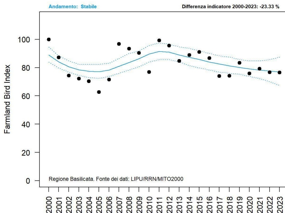
Figura 4. Andamento del Farmland Bird Index regionale nel periodo 2000-2023. I punti indicano i valori annuali del Farmland Bird Index (calcolato come media geometrica degli andamenti delle singole specie), la linea continua e le linee tratteggiate rappresentano rispettivamente la tendenza dell'indicatore ed il relativo intervallo di confidenza al 95% (stimati con MSIttools).
