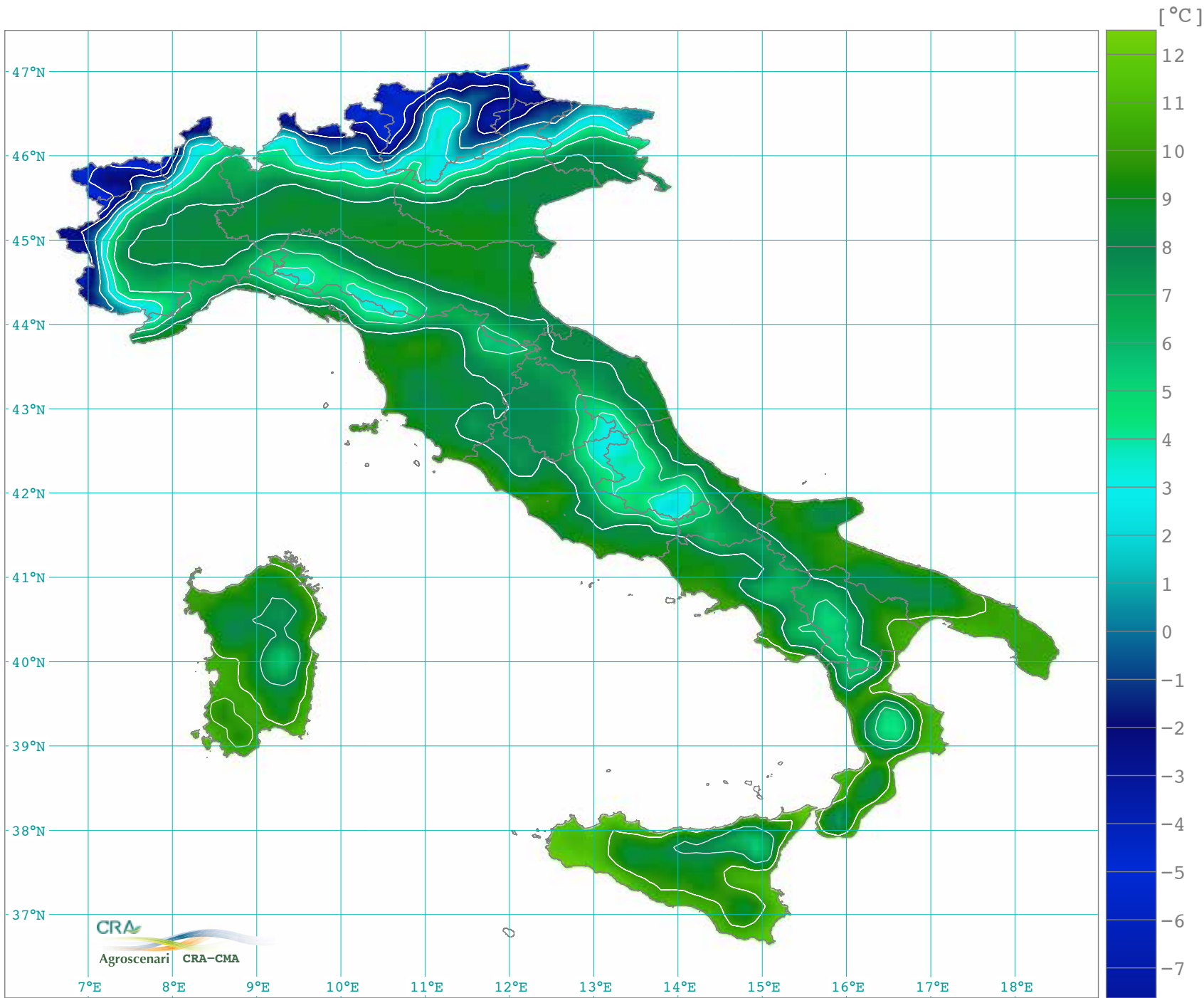
Temperatura minima media stagionale primavera: marzo, aprile e maggio (1961-1990)
