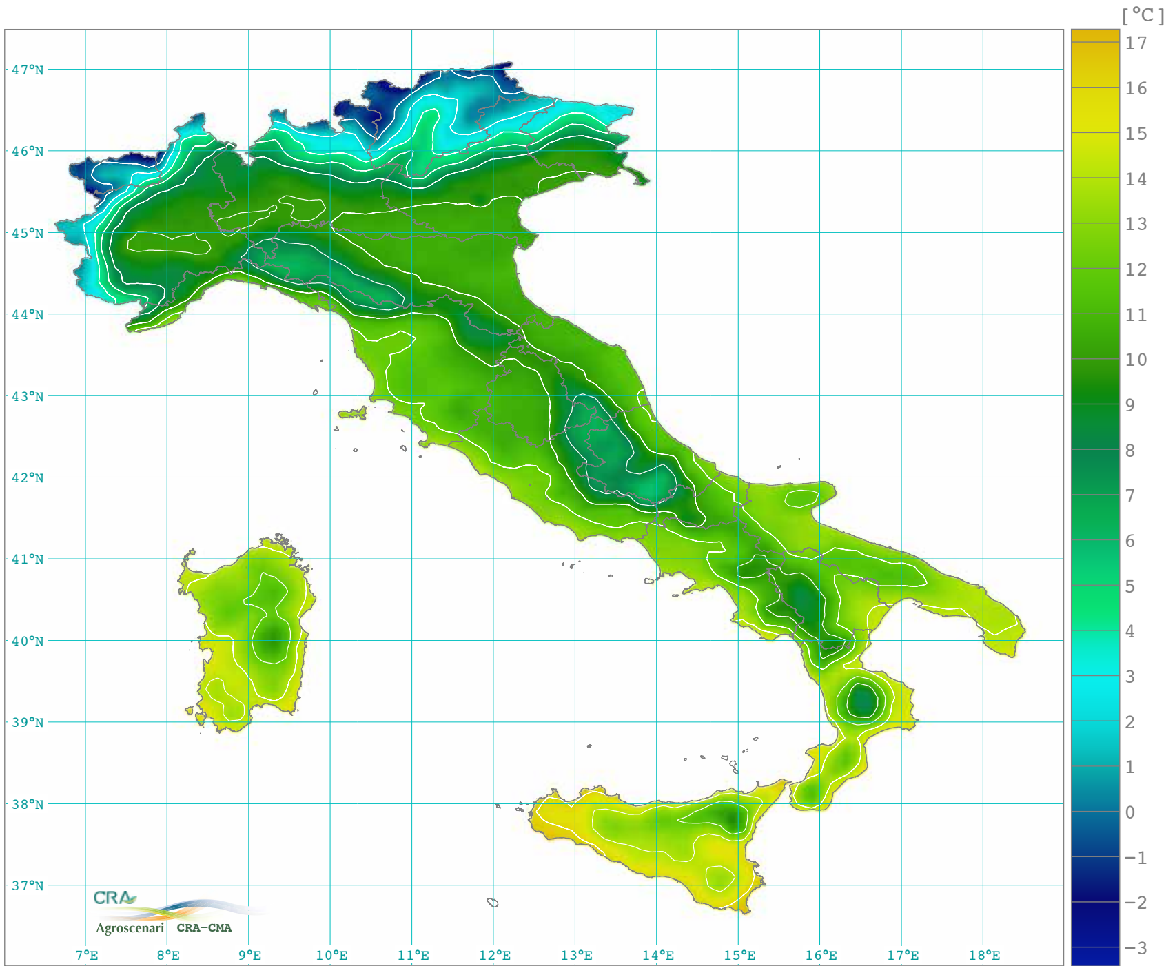
Temperatura minima media stagionale autunno: settembre, ottobre e novembre (1961-1990)
