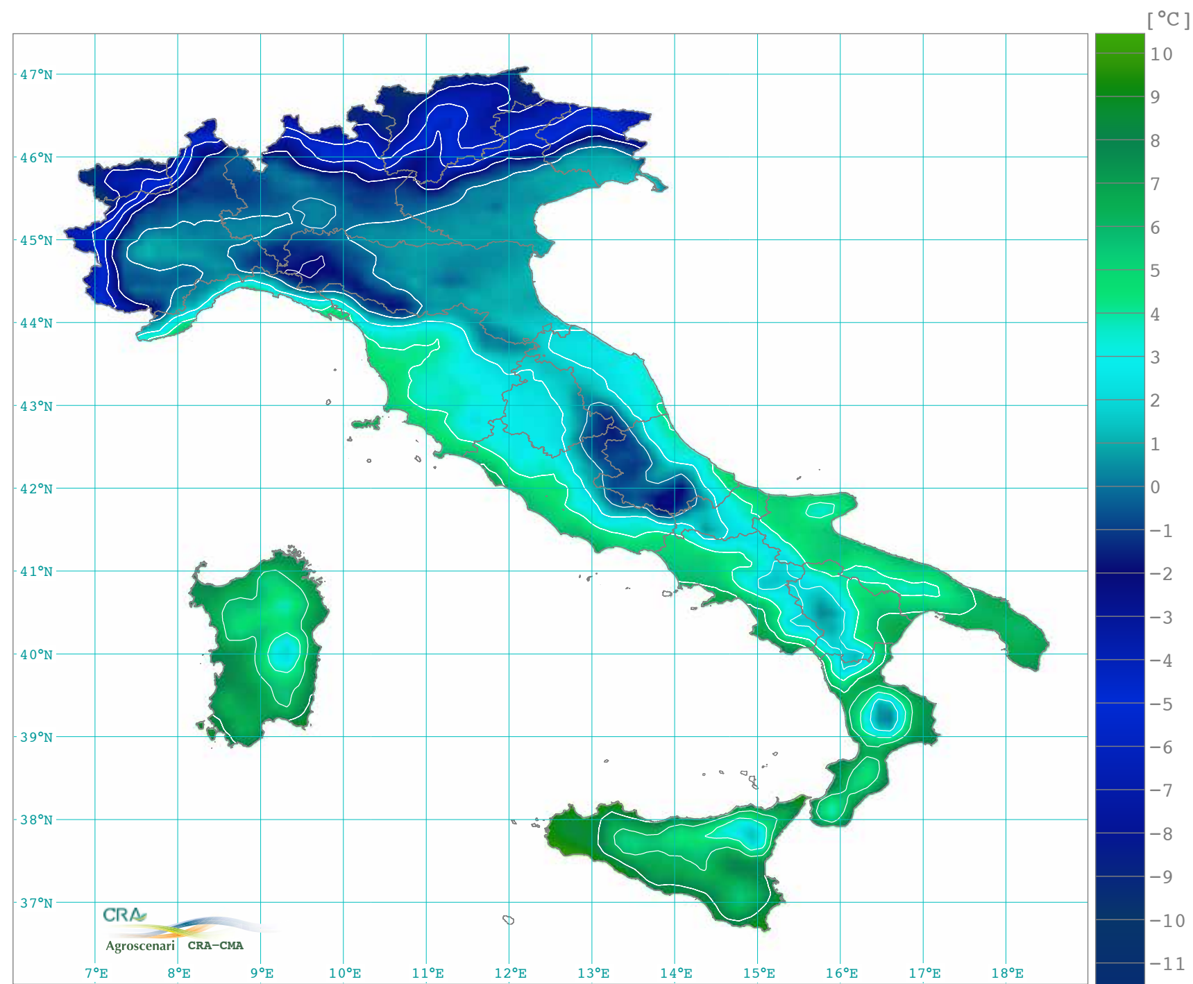
Temperatura minima media stagionale inverno: dicembre, gennaio e febbraio (1961-1990)
