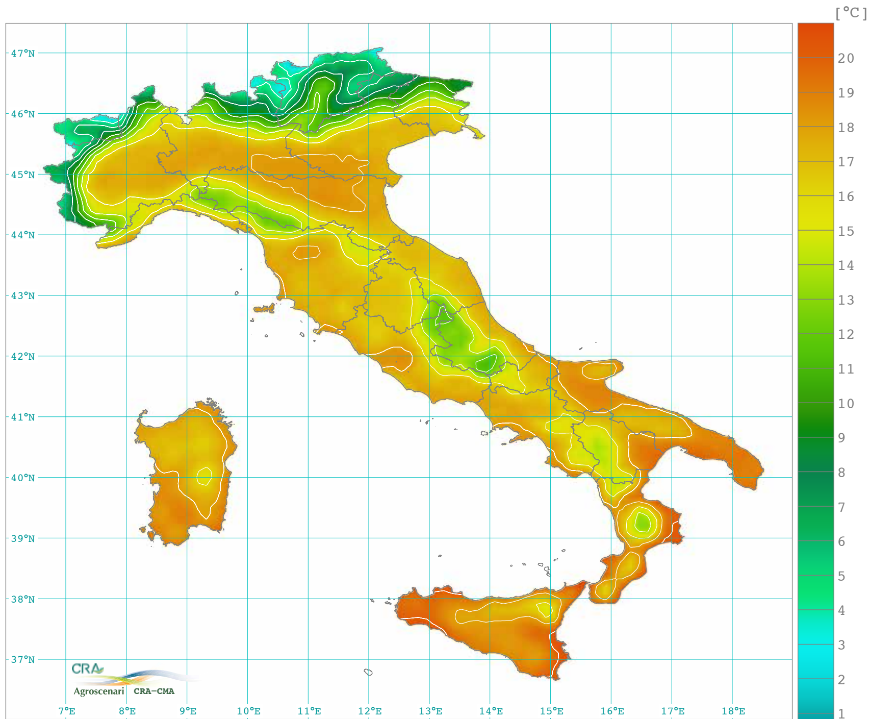
Temperatura minima media stagionale estate: giugno, luglio e agosto (1961-1990)
