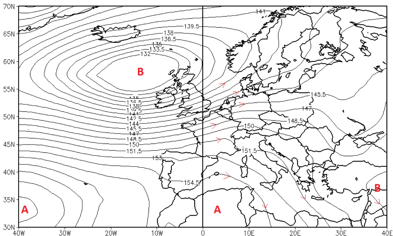
Fig. 1 - Topografia media del livello di pressione di 850 hPa (in media 1.5 km di quota) per il periodo 26 Luglio - 1 Agosto. Le frecce inserite danno un'idea orientativa della direzione e del verso del flusso, di cui considerano la sola componente geostrofica. Gli assi delle saccature sono in blu e quelli dei promontori in rosso.
