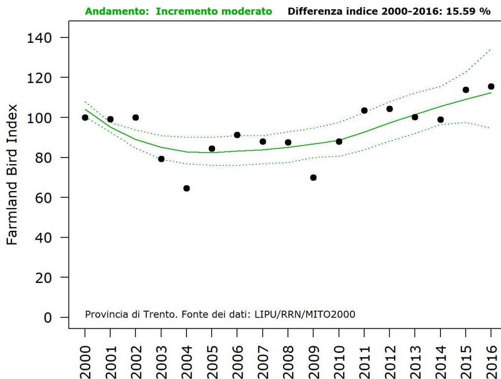
Figura 3.1: Andamento del Farmland Bird Index provinciale nel periodo 2000-2016. I punti indicano i valori annuali del Farmland Bird Index (calcolato come media geometrica degli andamenti delle singole specie), la linea continua e le linee tratteggiate rappresentano rispettivamente la tendenza dell'indice ed il relativo intervallo di confidenza al 95% (stimati con MSI-tool).
