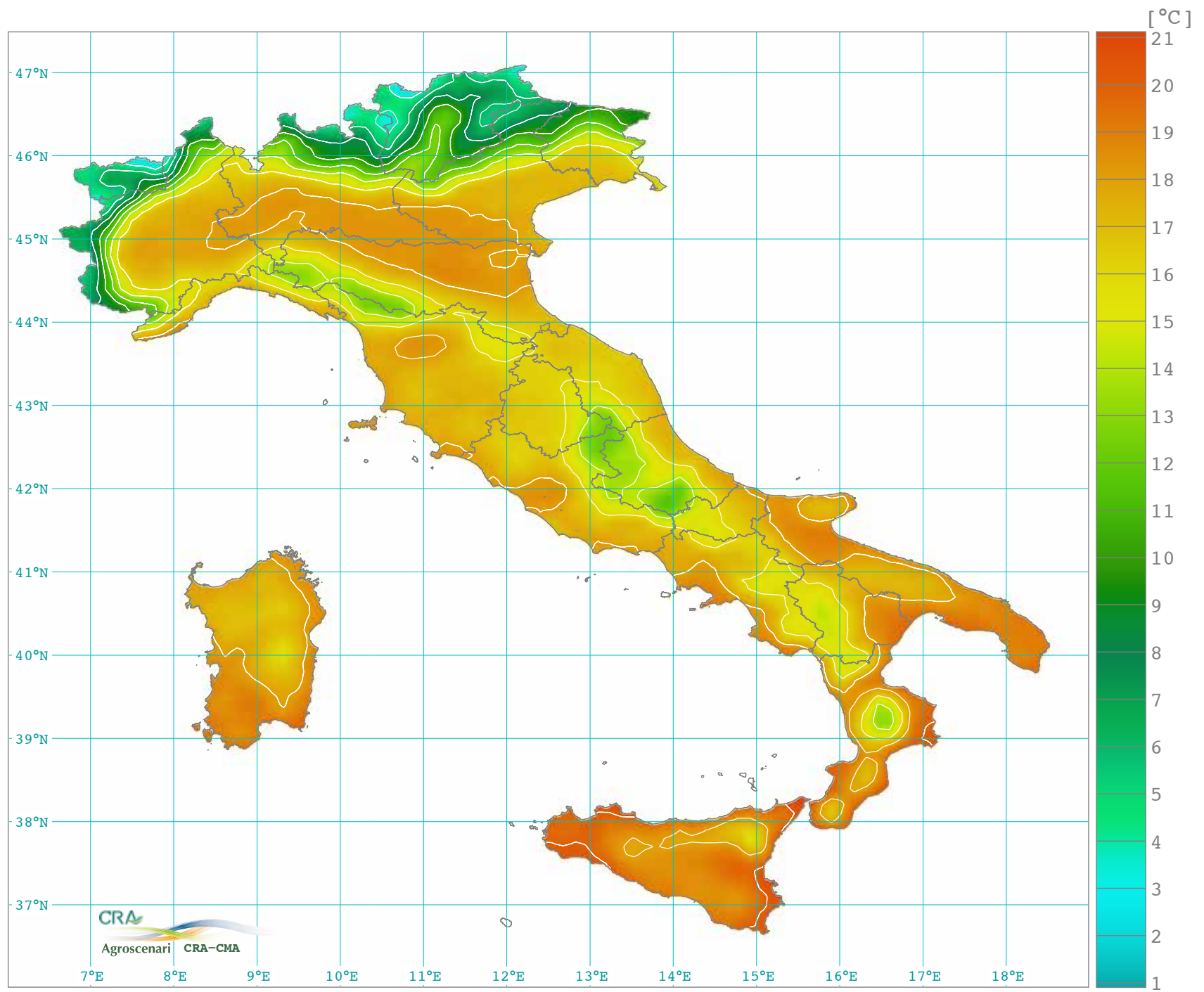
Temperatura minima media stagionale estate: giugno, luglio e agosto (1971-2000)
