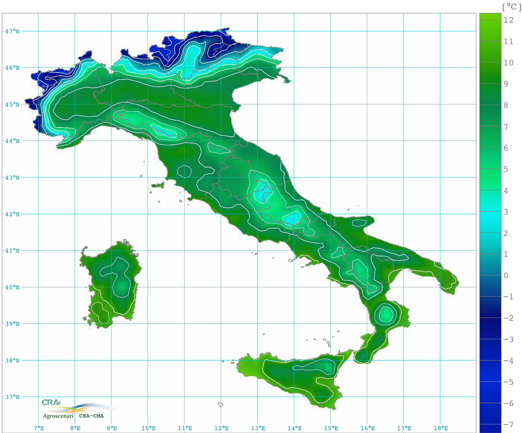
Temperatura minima media stagionale primavera: marzo, aprile e maggio (1971-2000)
