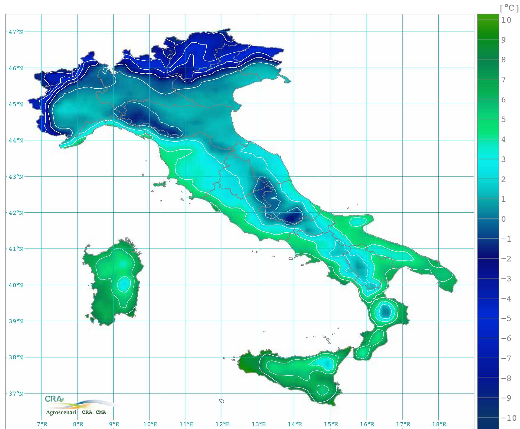
Temperatura minima media stagionale inverno: dicembre, gennaio e febbraio (1971-2000)
