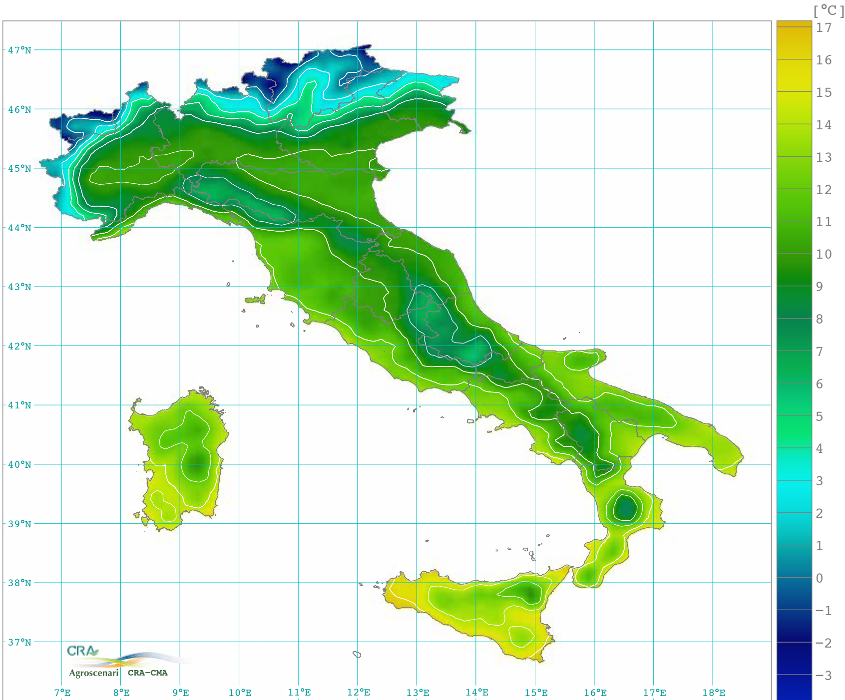
Temperatura minima media stagionale autunno: settembre, ottobre e novembre (1971-2000)
