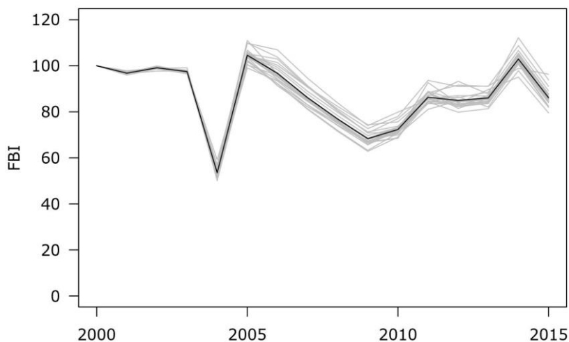
Figura 5: Farmland Bird Index provinciale nella sua versione definitiva (linea nera) e nelle versioni risultanti dal ricalcolo dell'indicatore effettuato togliendo di volta in volta una delle specie agricole.
