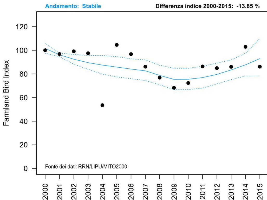
Figura 3: Andamento del Farmland Bird Index provinciale nel periodo 2000-2015. I punti indicano i valori annuali del Farmland Bird Index (calcolato come media geometrica degli andamenti delle singole specie), la linea continua e le linee tratteggiate rappresentano rispettivamente la tendenza dell'indice ed il relativo intervallo di confidenza al 95% (stimati con MSI-tool).
