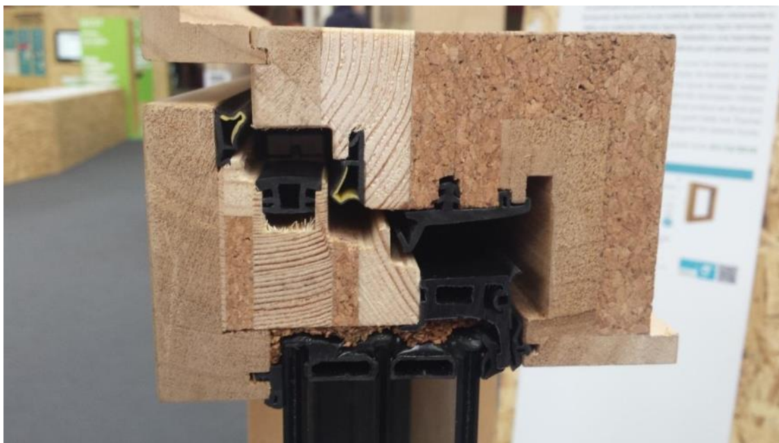
Figura 6.4 – Esempio di strato isolante in sughero per un infisso (foto Romagnoli)
