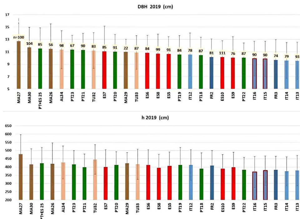
Figura 2.7 – Confronto tra altezze (h) e diametri a petto d’uomo (DBH) di 27 provenienze “mediterranee” al ventesimo anno di età in Sardegna (le iniziali indicano i paesi di provenienza: MA Marocco, AL Algeria, TU Tunisia, etc., il numero apicale su ogni istogramma il numero di piante in prova) (Fernández Paradela et al. 2019).
