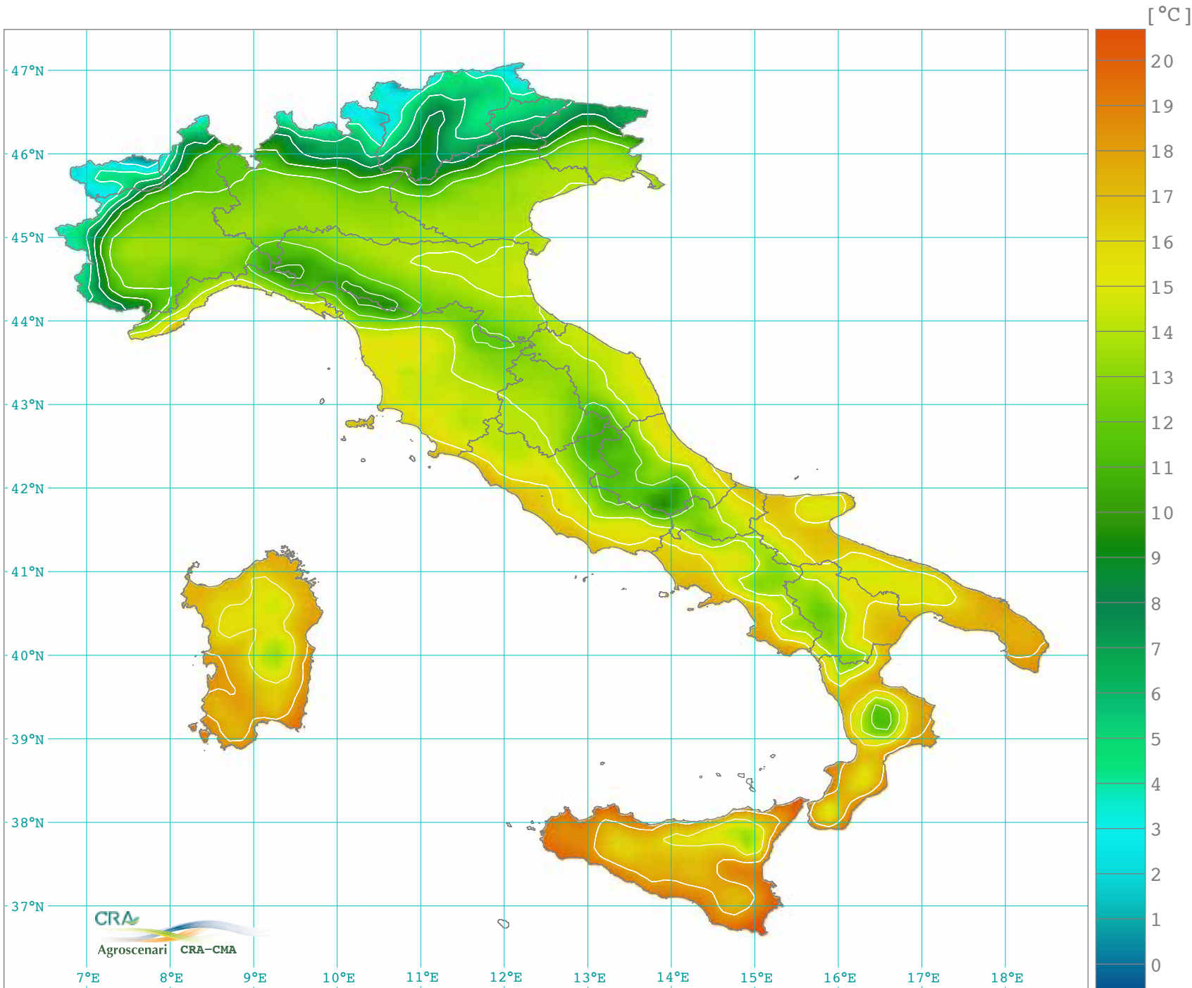
Temperatura media stagionale autunno: settembre, ottobre e novembre (1971-2000)
