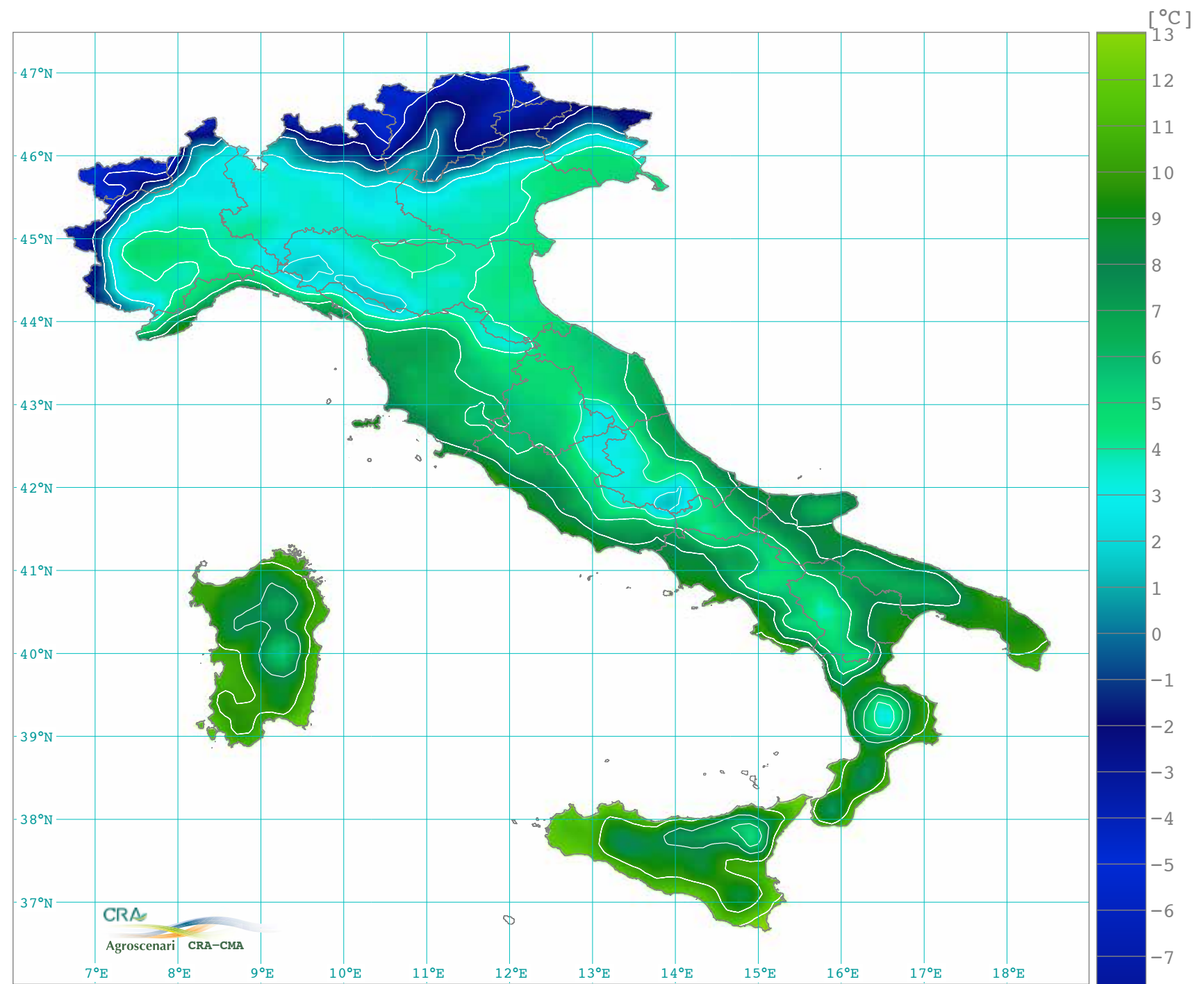
Temperatura media stagionale inverno: dicembre, gennaio e febbraio (1971-2000)
