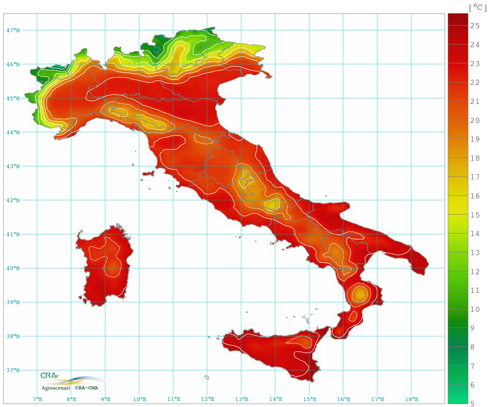
Temperatura media stagionale estate: giugno, luglio e agosto (1971-2000)
