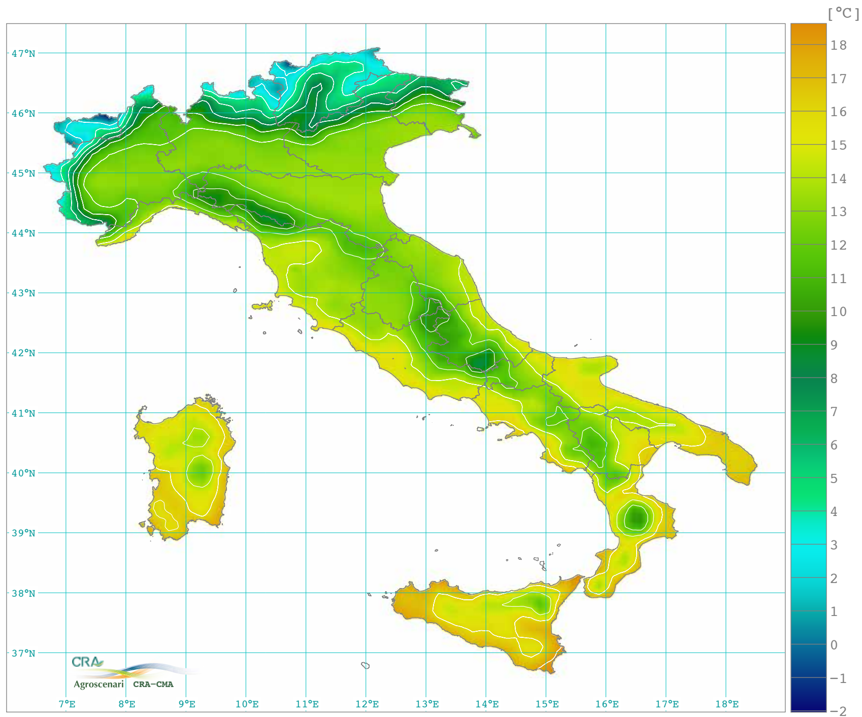
Temperatura media annua (1971-2000)
