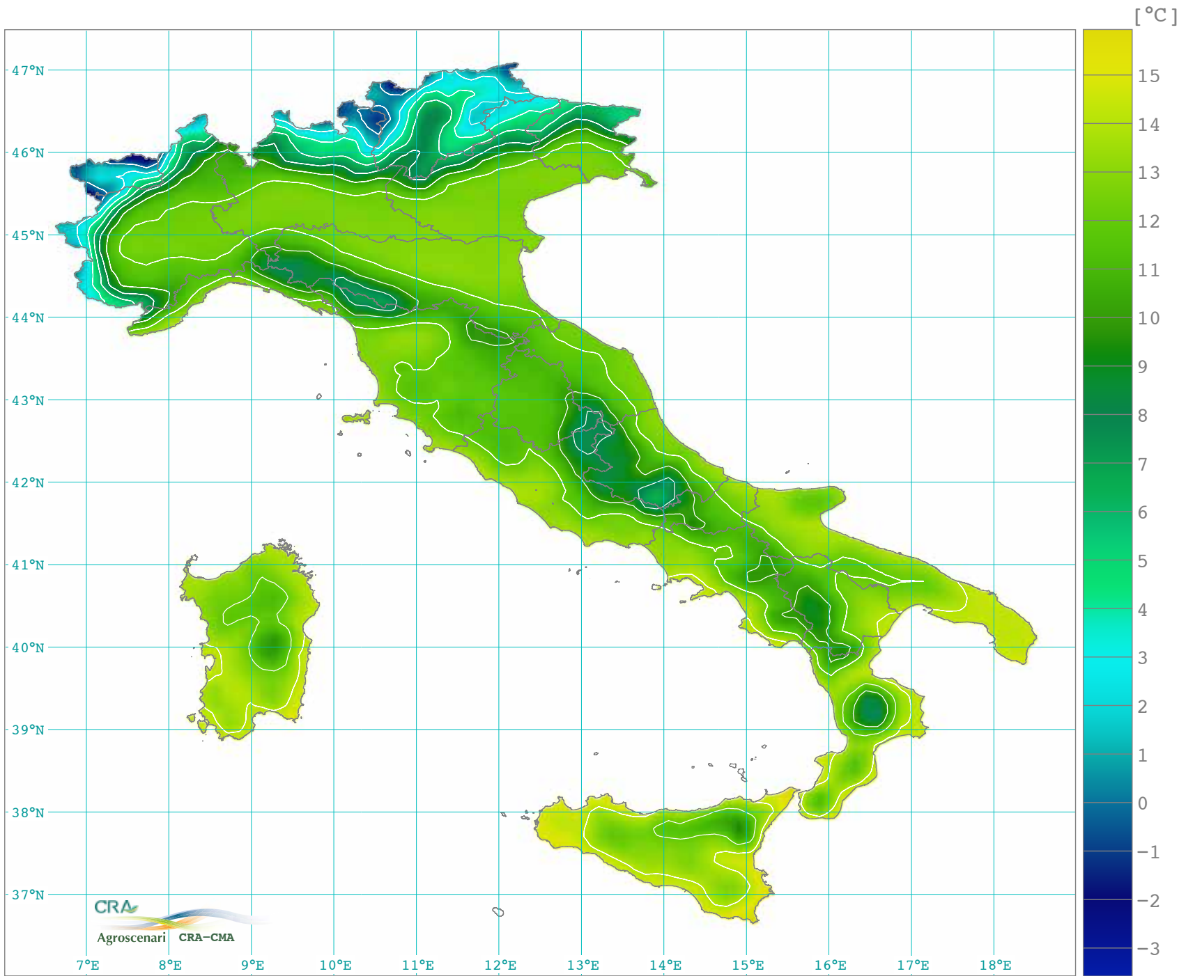
Temperatura media stagionale primavera: marzo, aprile e maggio (1971-2000)
