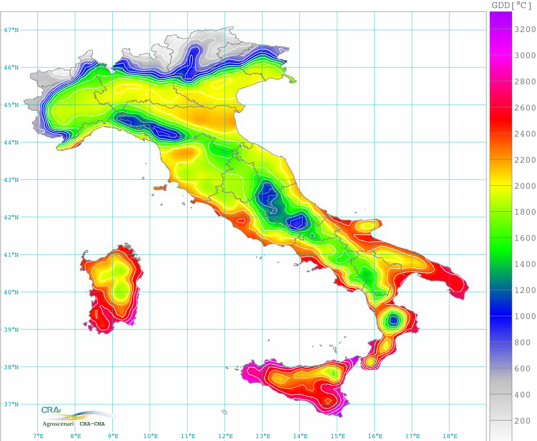
Somma termiche annue soglia 10 °C (1981-2010)
