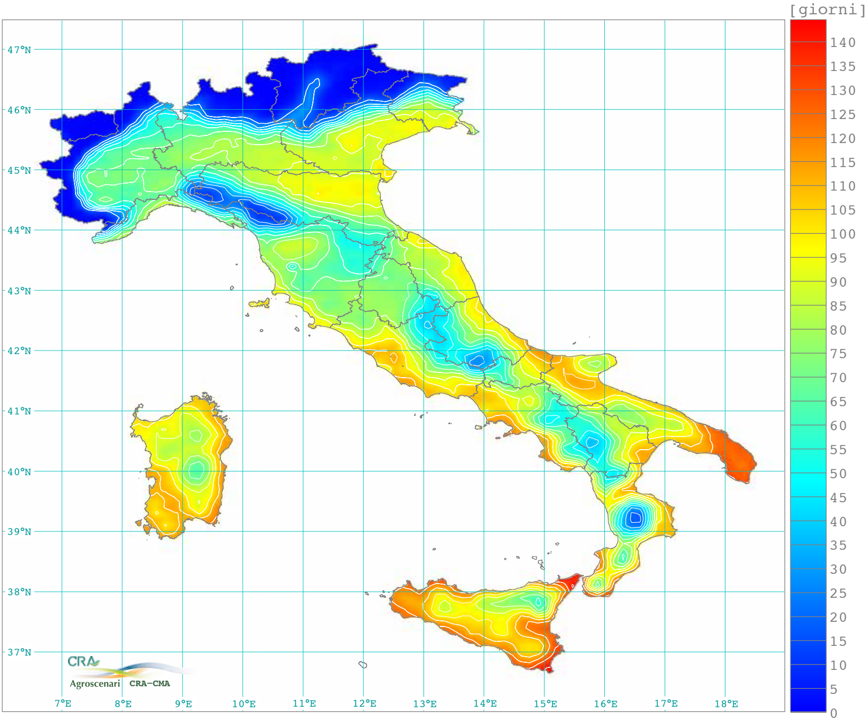
Numero medio annuo di giorni estivi (1981-2010)
