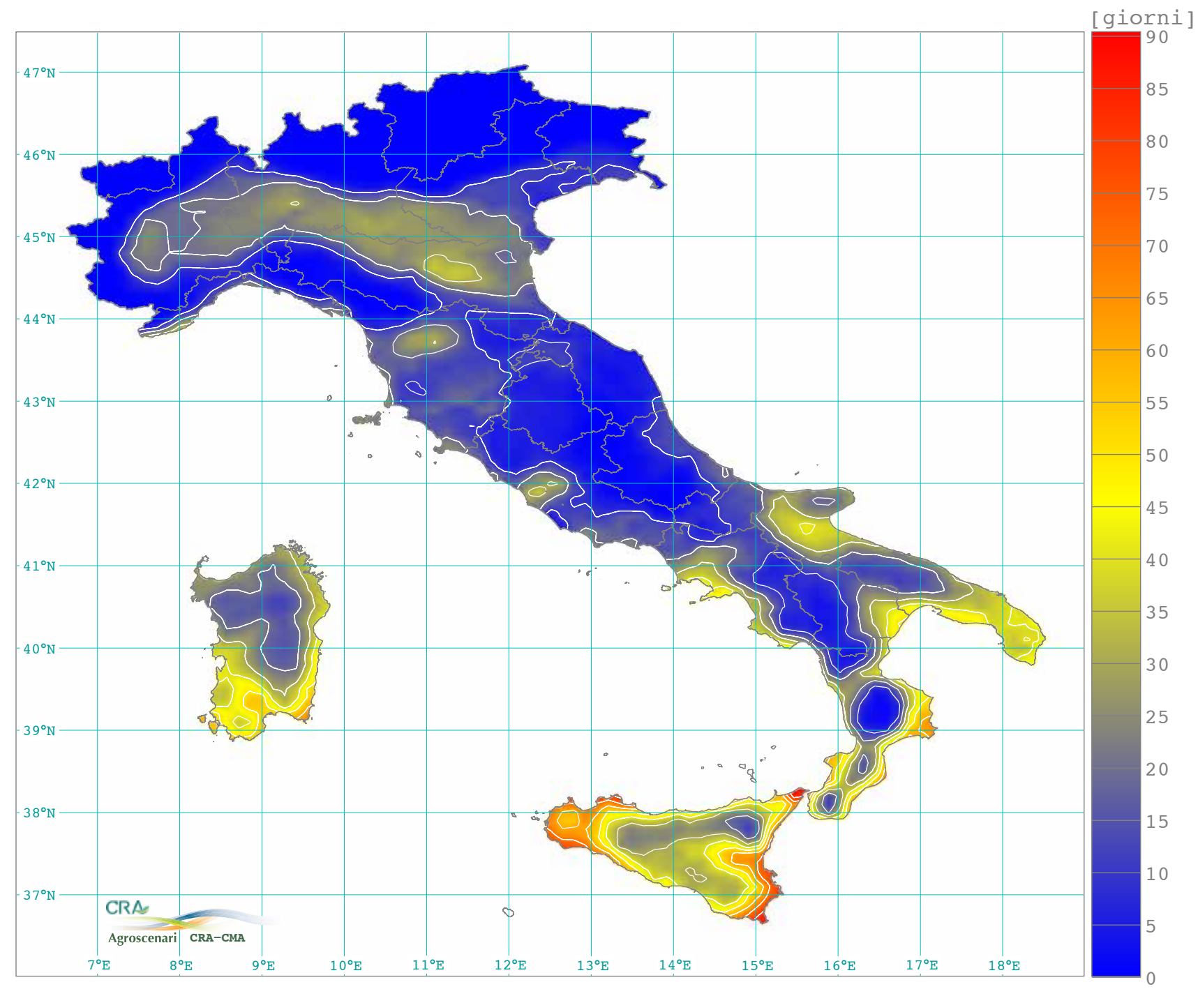
Numero medio annuo di notti tropicali (1981-2010)
