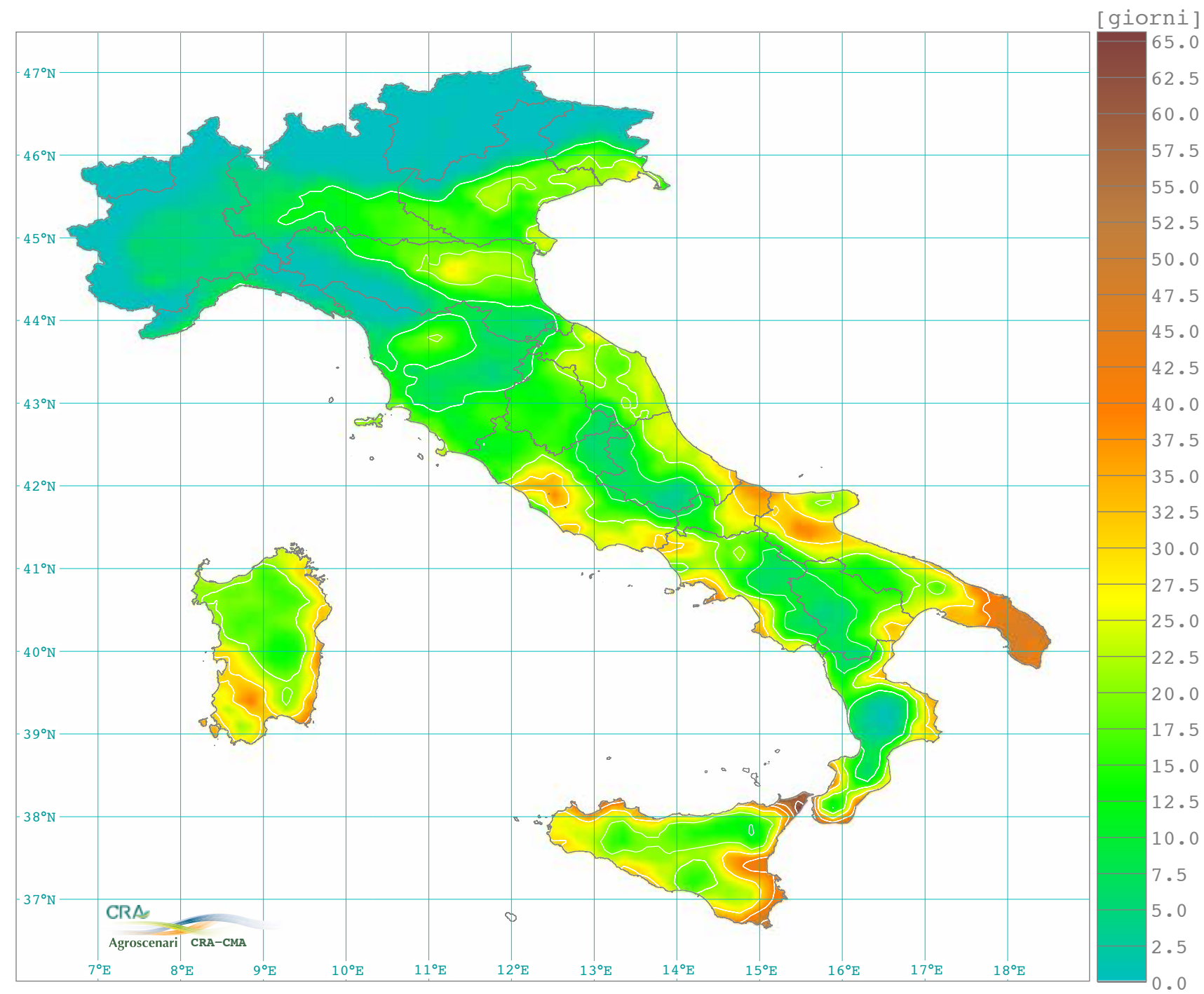
Numero medio annuo di giorni con temperatura massima > 30 °C (1981-2010)
