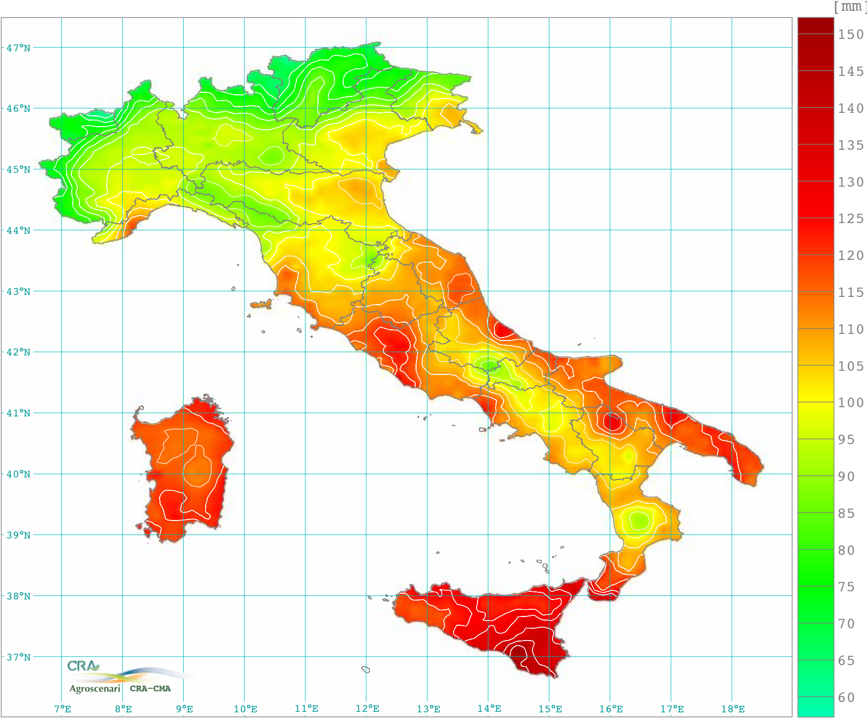
Evapotraspirazione potenziale totale agosto (1981-2010)
