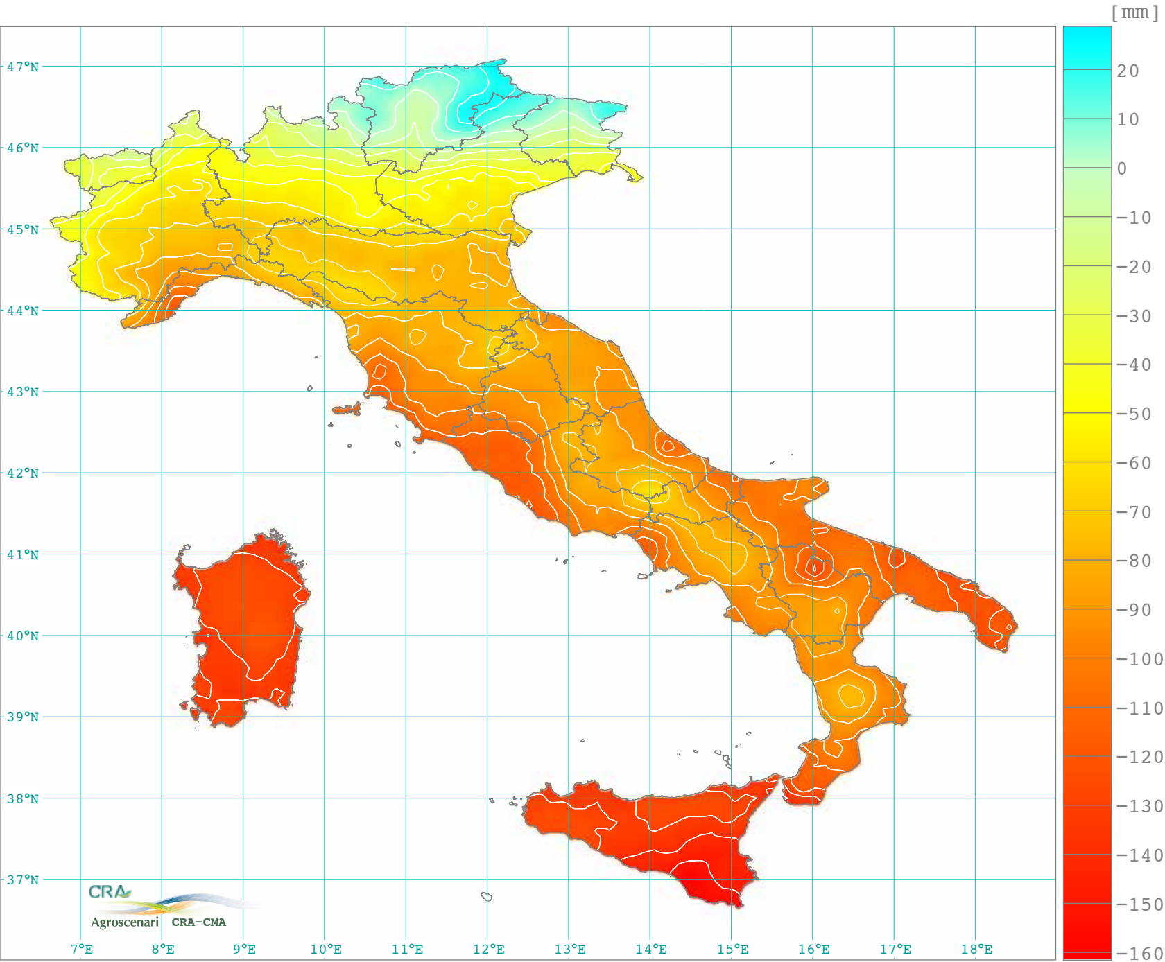
Bilancio idroclimatico mensile luglio (1981-2010)
