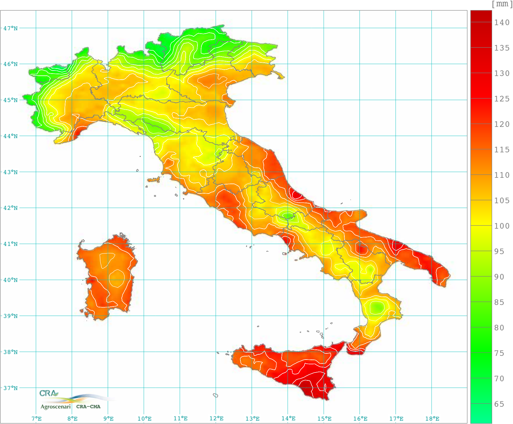
Evapotraspirazione potenziale totale giugno (1981-2010)
