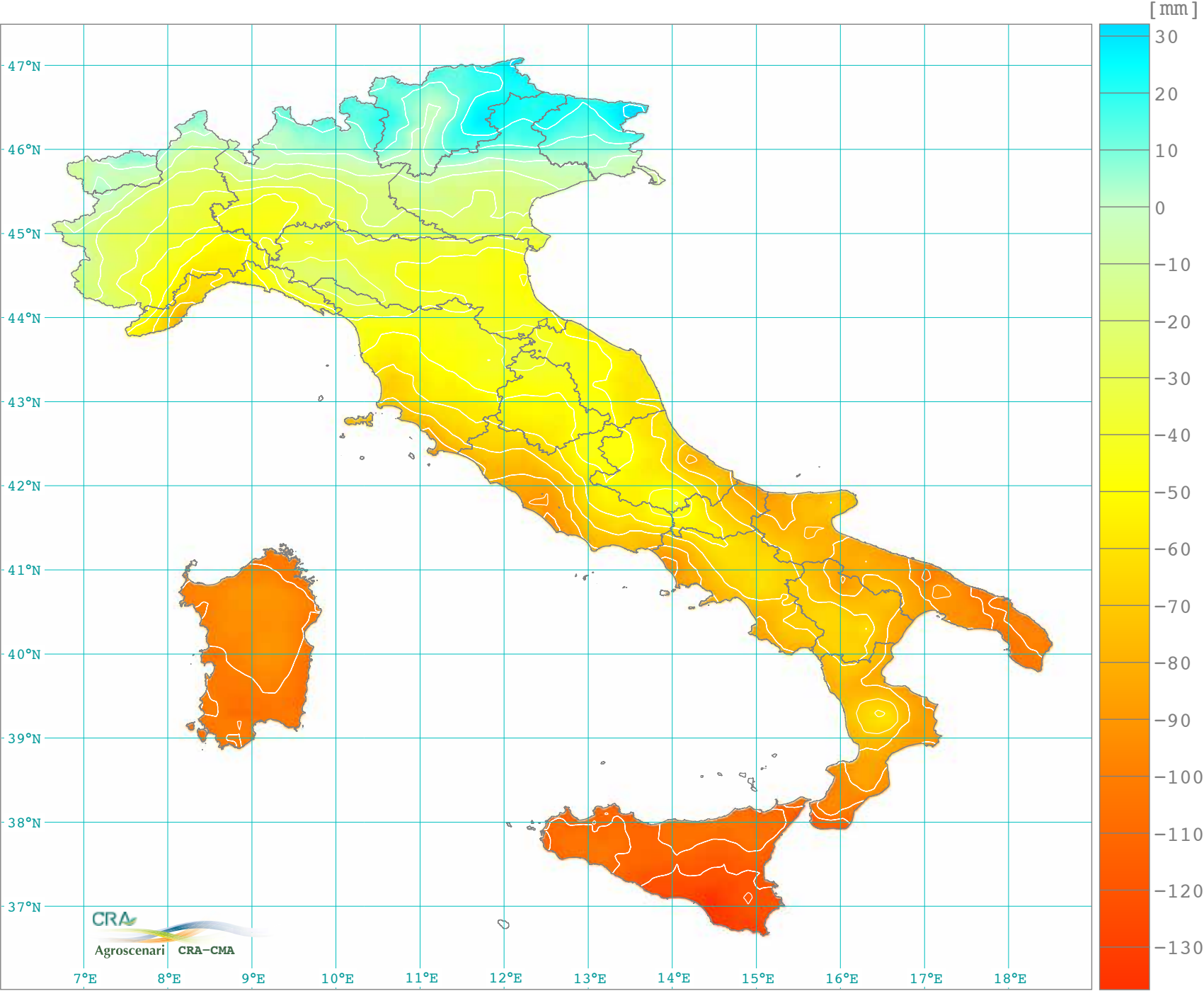
Bilancio idroclimatico mensile giugno (1981-2010)
