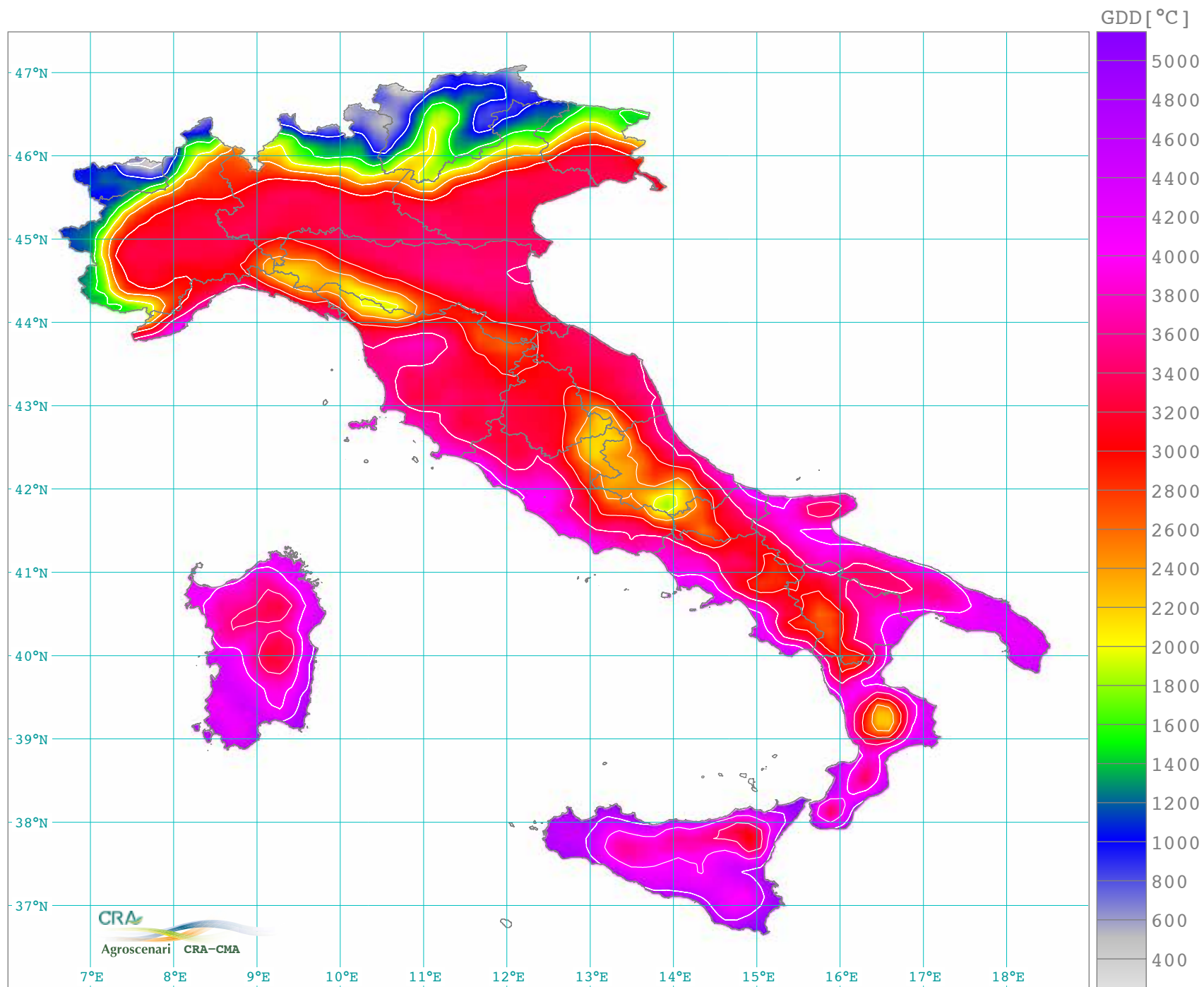
Sommatorie termiche annue soglia 5 °C (1981-2010)
