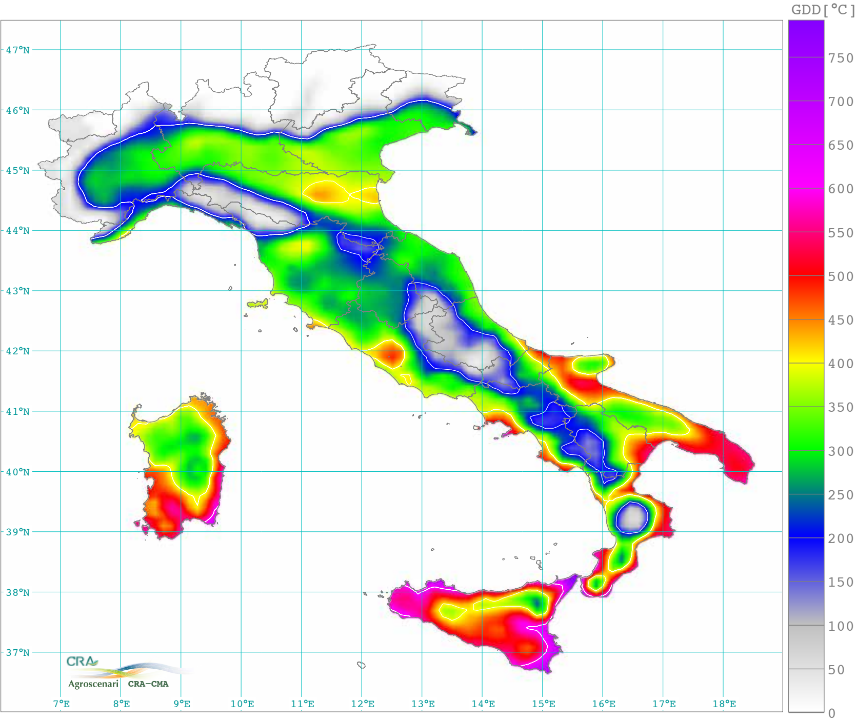
Sommatorie termiche annue soglia 20 °C (1981-2010)
