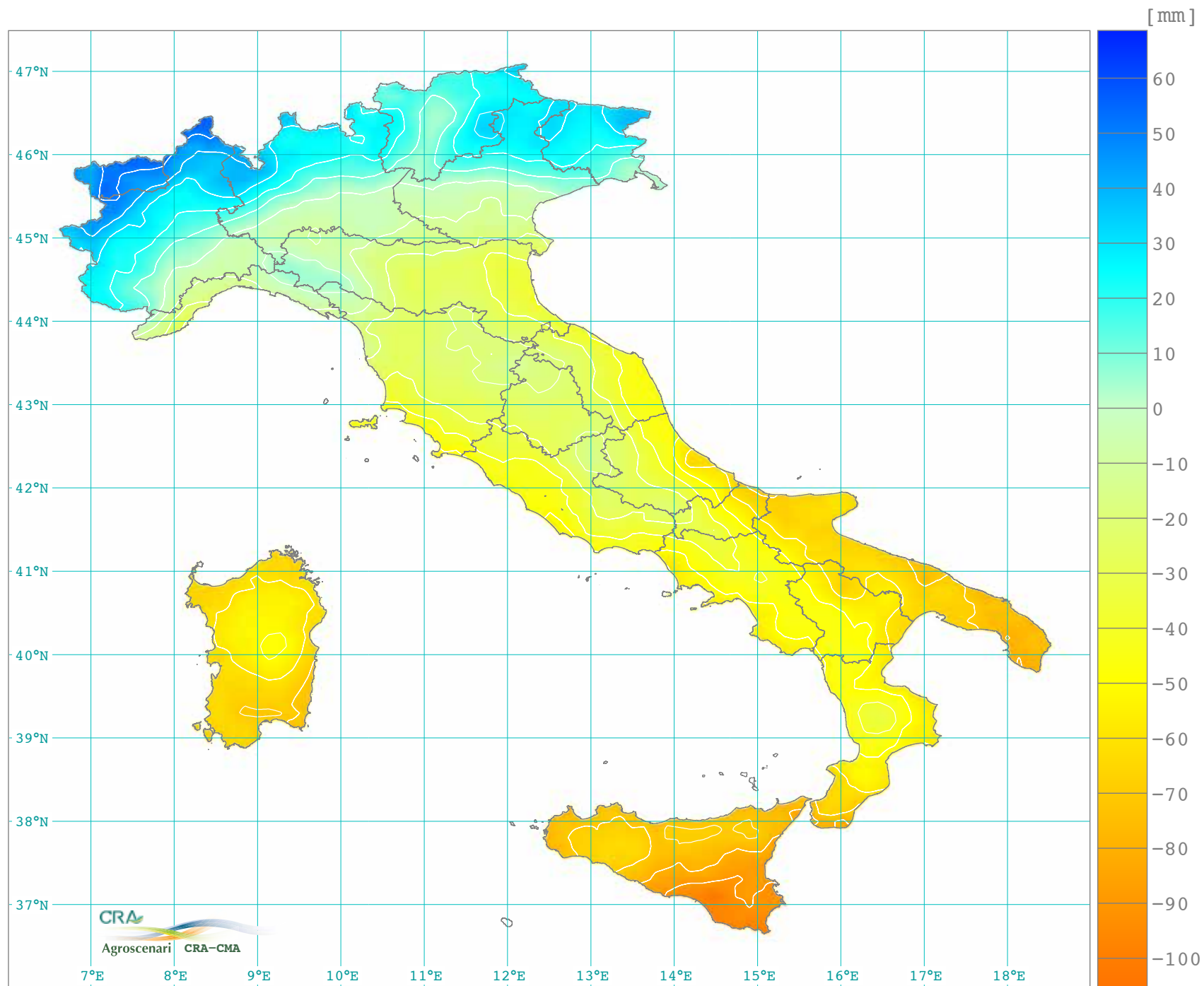
Bilancio idroclimatico mensile maggio (1981-2010)
