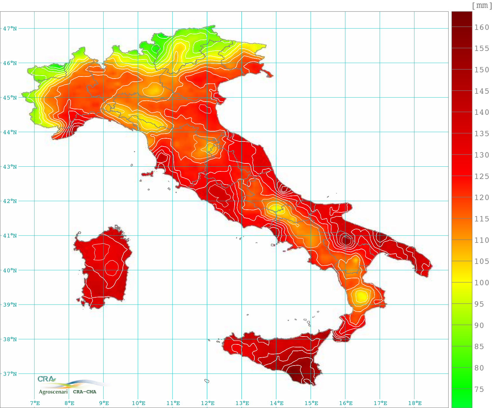
Evapotraspirazione potenziale totale luglio (1981-2010)
