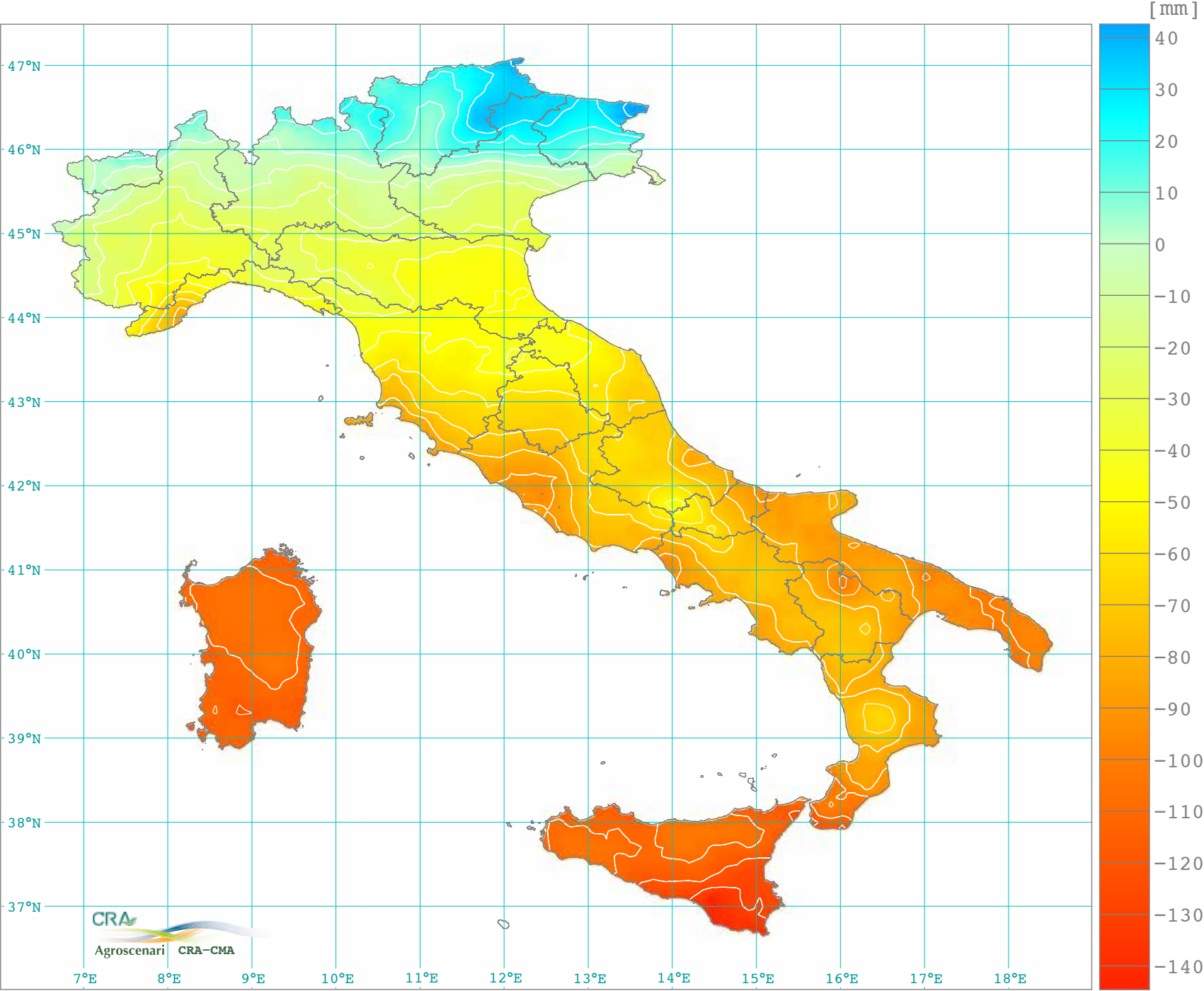
Bilancio idroclimatico mensile agosto (1981-2010)
