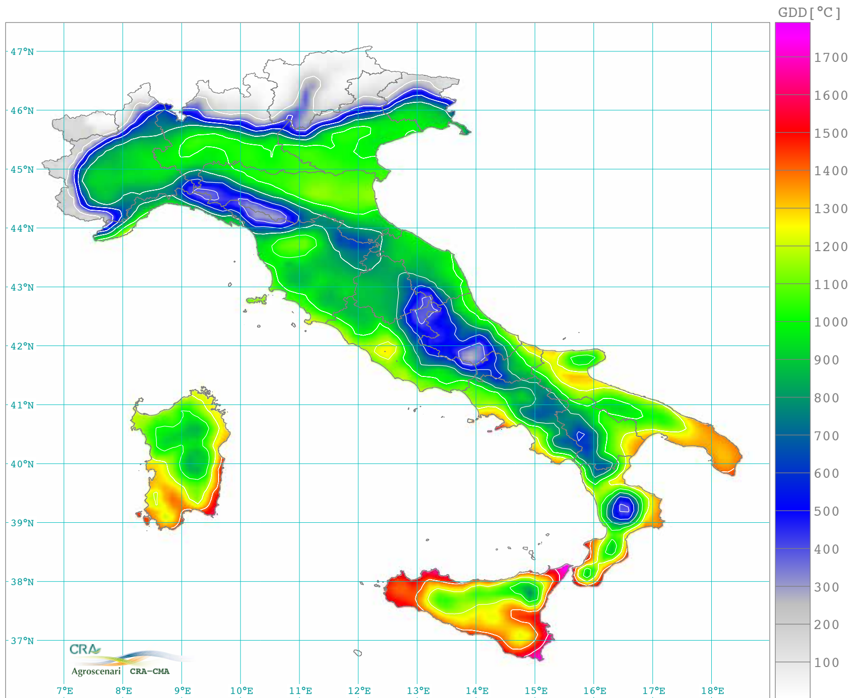
Sommatorie termiche annue soglia 15 °C (1981-2010)
