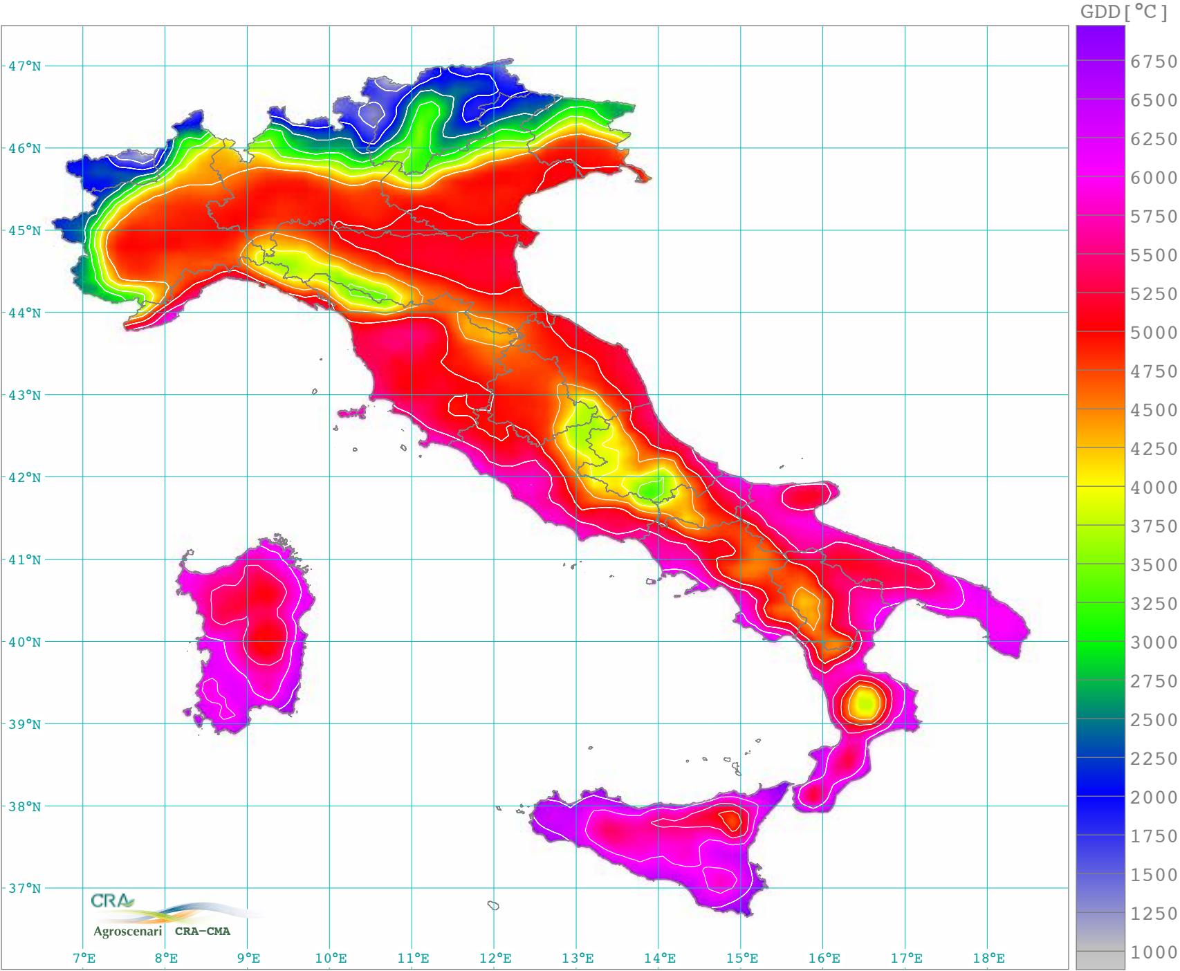
Somma termiche annue soglia 0 °C (1981-2010)
