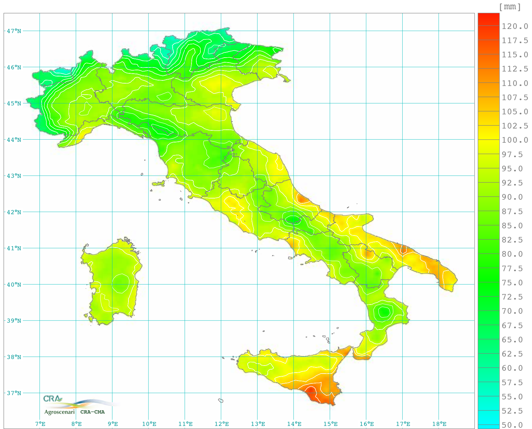
Evapotraspirazione potenziale totale maggio (1981-2010)
