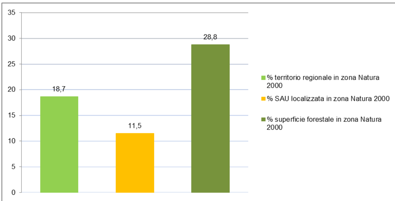
Figura 4.9 Aree Natura 2000 – incidenza sul territorio, sulla SAU e sulla superficie forestale - Fonte: Elaborazione su dati Eurostat (ICC34) – Aree Natura 2000 - Anno 2011
