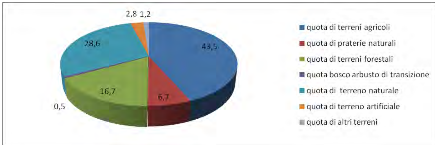
Figura 4.8 Copertura del suolo per tipologia presente in Sardegna (% del totale della superficie)-Fonte: elaborazione su dati Eurostat – (ICC31)-Copia del suolo - Anno – 2006
