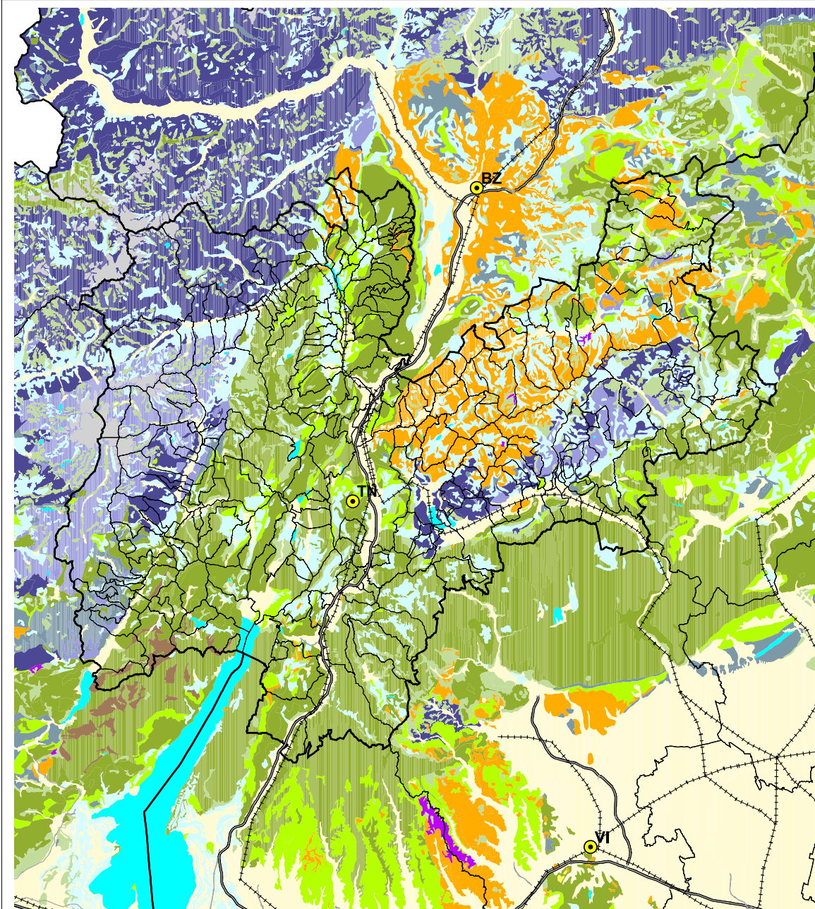
fig. 3c - Litologia
