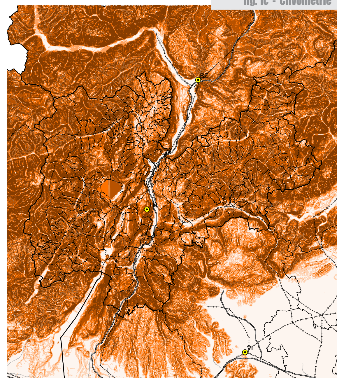
Carta clivometrica
