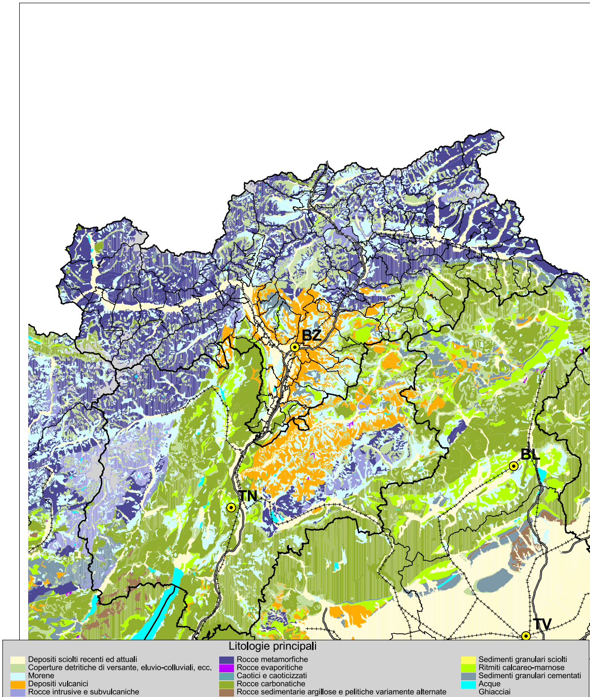
fig. 3c - Litologia
