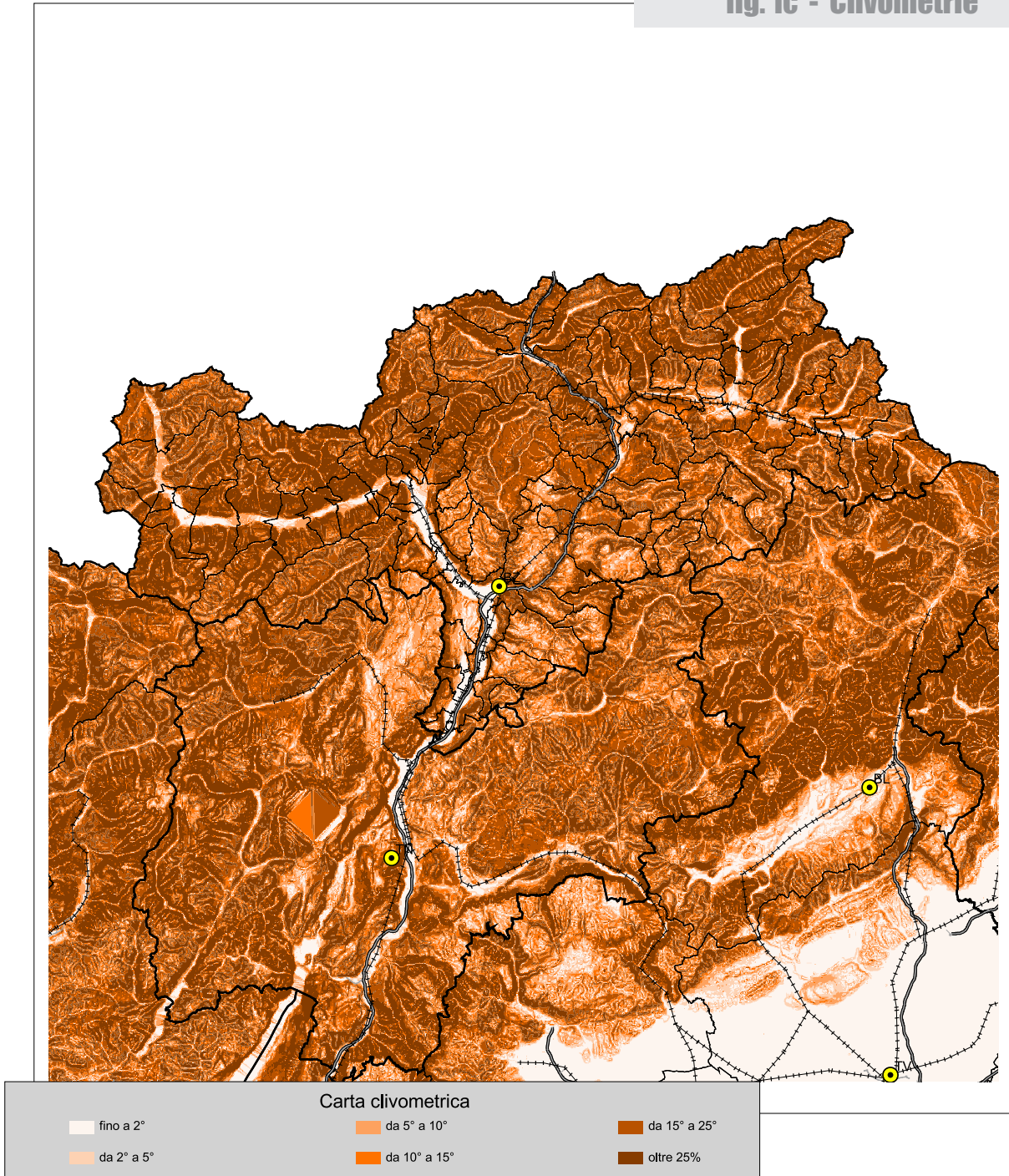
fig. 1c - Clivometrie
