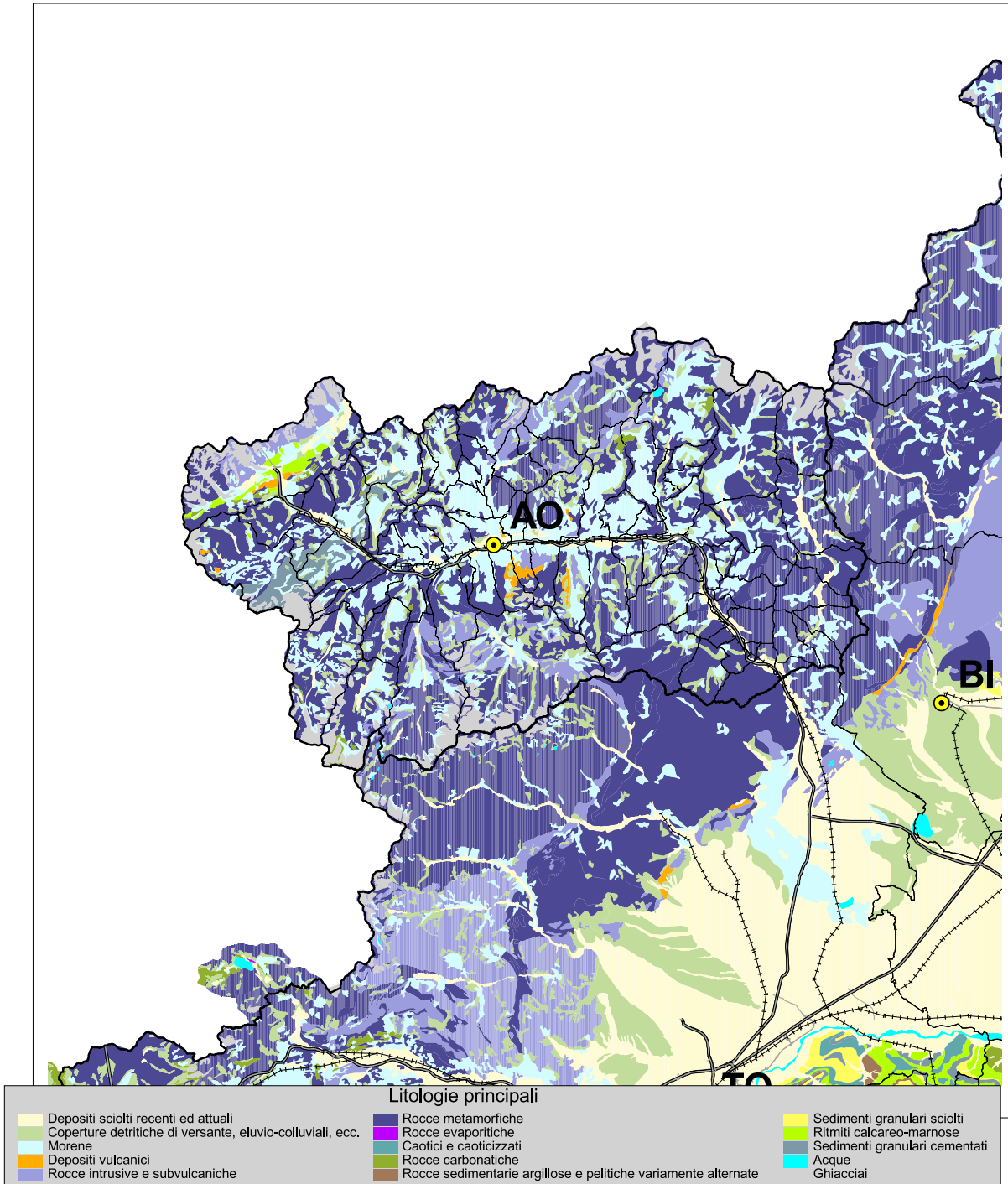
fig. 3c - Litologia
